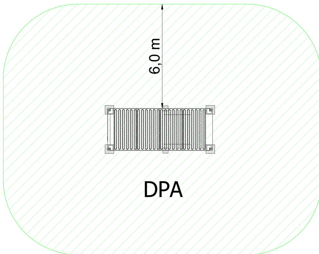
Figura 4.5 - DPA per le Cabine di conversione e trasformazione
