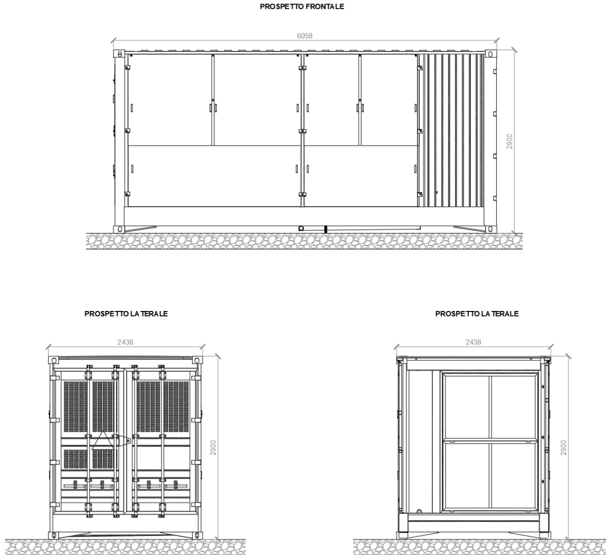
Figura 4.4 - Tipologia cabinati metallici per cabina di conversione/trasformazione – dimensioni in mm
