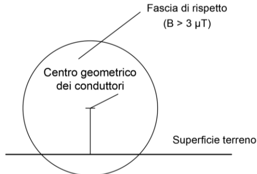
Figura 2.1 - Fascia di rispetto intorno all'elettrodotto
