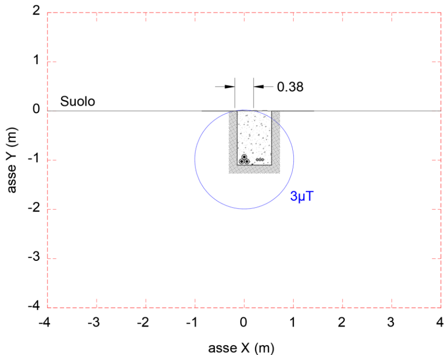
Figura 4.1 - Curva Equilivello 3 μT – 1 terna di cavi a 36 kV
