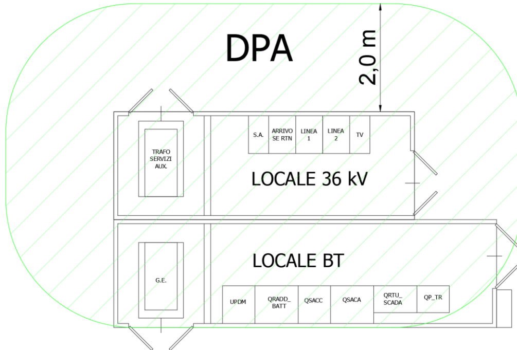
Figura 4.7 - DPA Cabina Elettrica Utente
