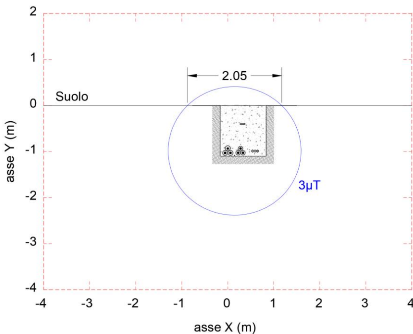
Figura 4.2 - Curva Equilivello 3μT – 2 terne di cavi a 36 kV
