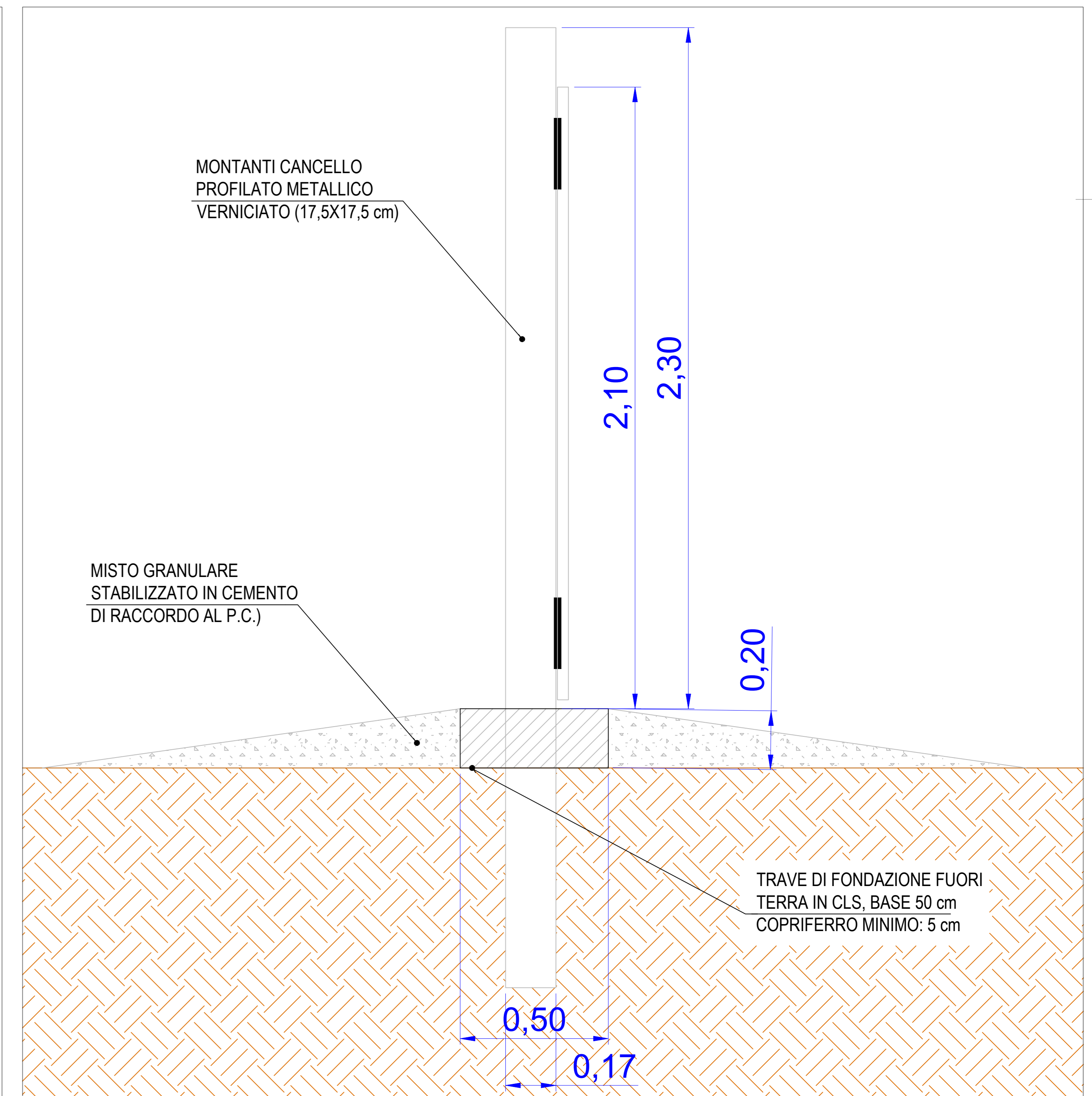
Recinzione - sezione Scala 1:10
