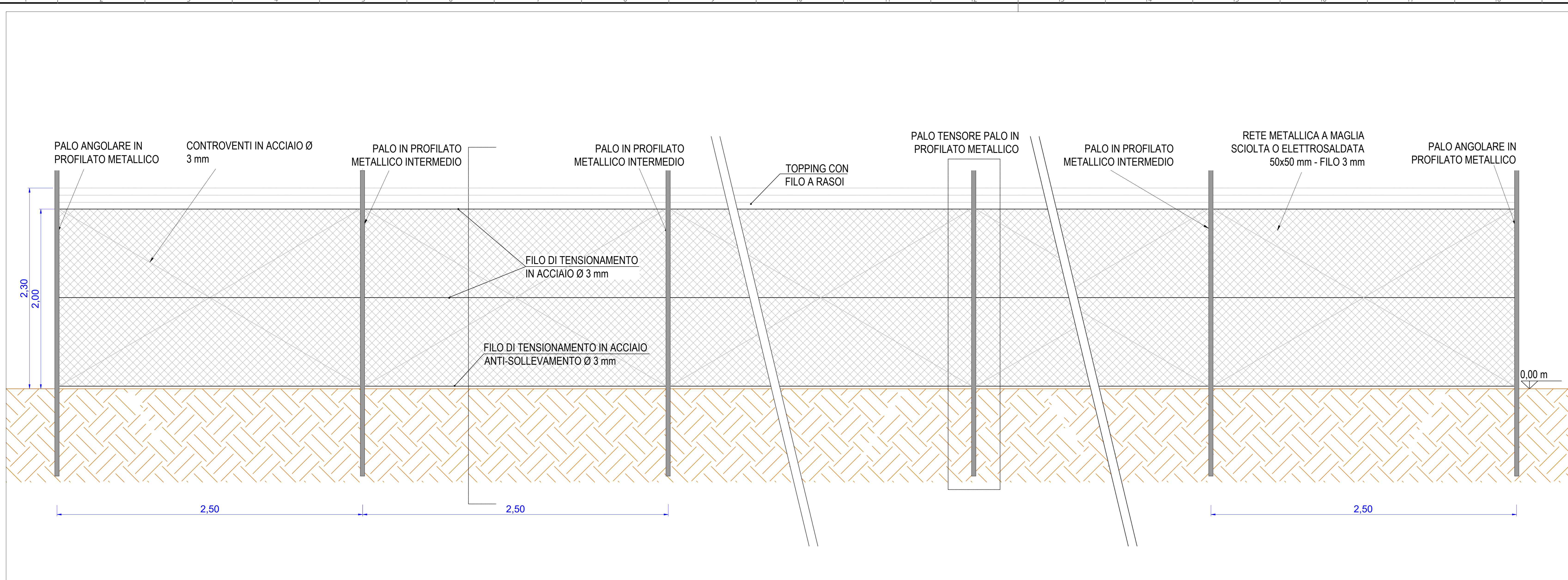
Recinzione - vista frontale Scala 1:20
