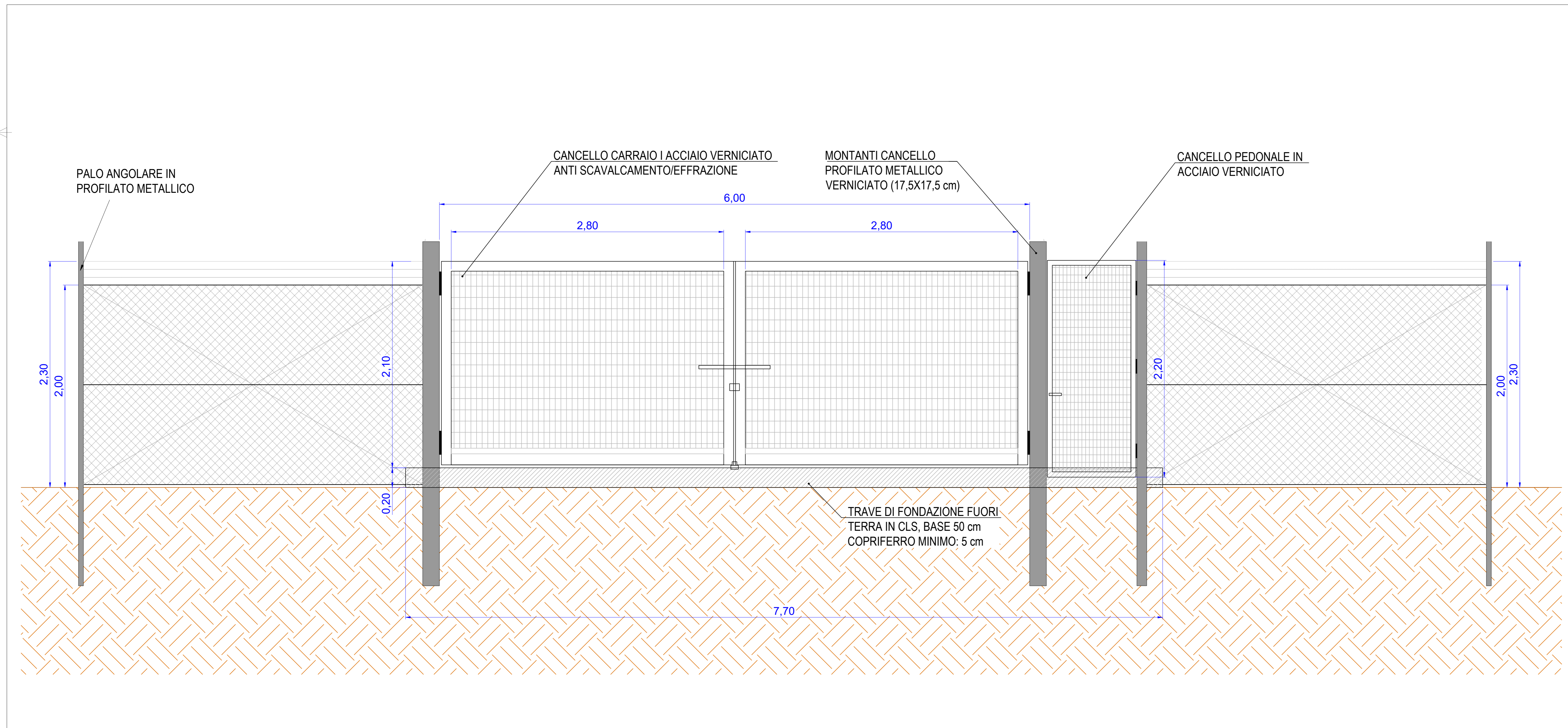
Cancello di accesso - vista frontale Scala 1:20
