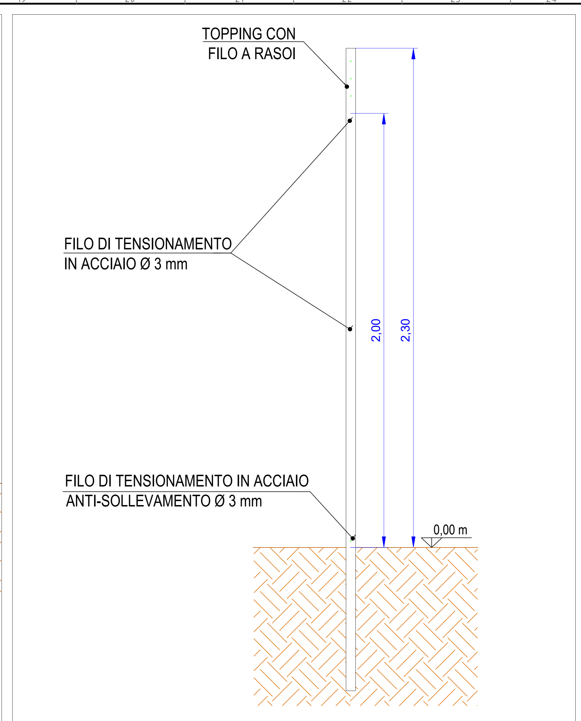
Recinzione - sezione Scala 1:10
