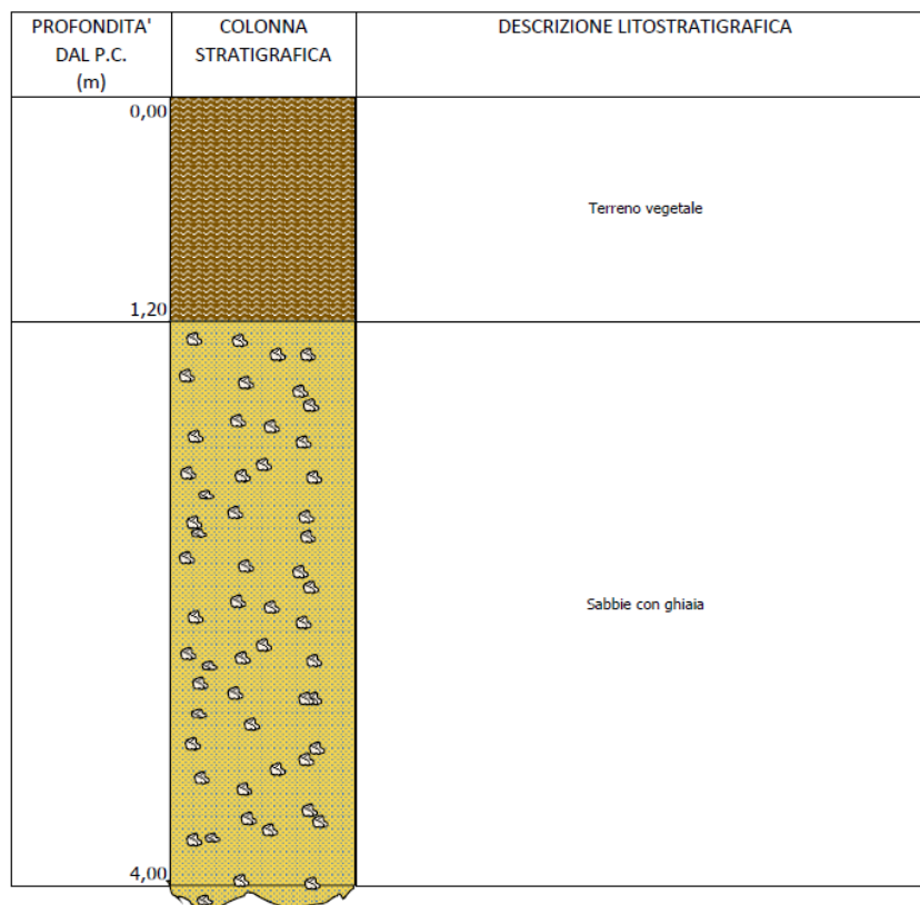
Fig. 5 – Colonna stratigrafica
