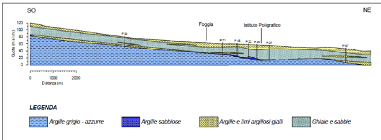
Fig. 4 – Sezione geolitologica del Tavoliere in corrispondenza del tratto medio-basso del bacino idrografico del Torrente Cervaro (da Sollitto, 2006)
