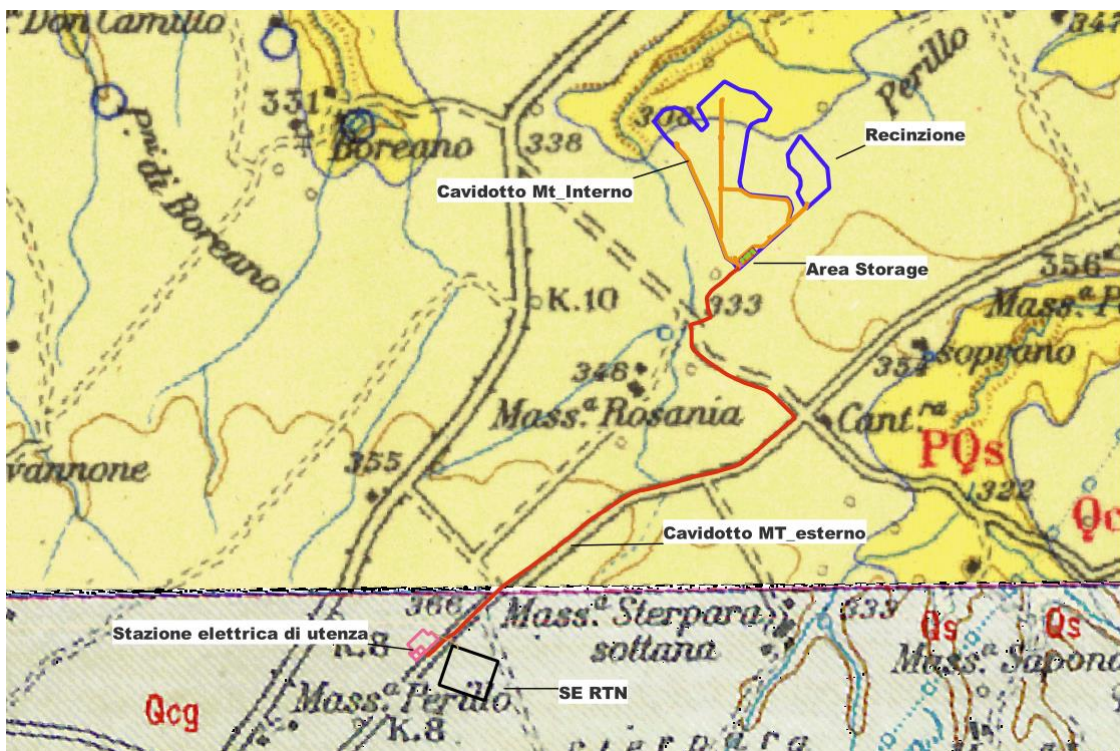
Figura 2 - Stralcio Carta Geologica d'Italia 1:100.000 Fogli n. 175 (Cerignola) e n. 187 Melfi della Carta Geologica d'Italia in scala 1:100.000
