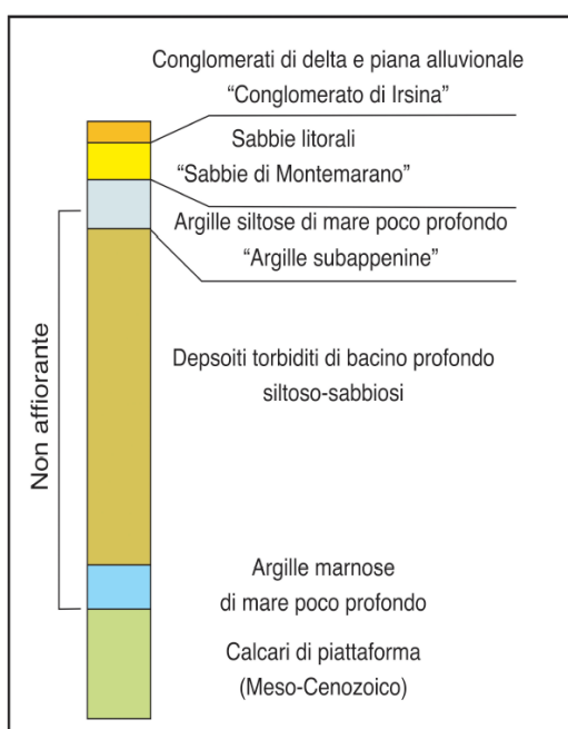
Figura 3 - Serie stratigrafica Bradanica
