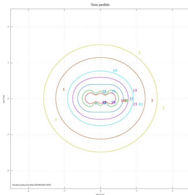
Figura 21: DPA tratto 5-4 (valori calcolati con l'ausilio del software Magic)
