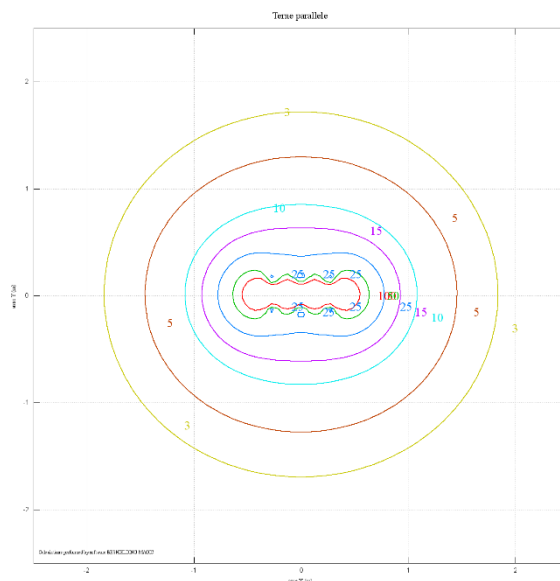
Figura 25: DPA tratto 2-1 (valori calcolati con l'ausilio del software Magic)
