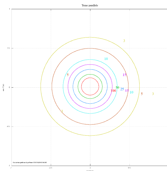
Figura 11: DPA tratto T08-8 (valori calcolati con l'ausilio del software Magic)
