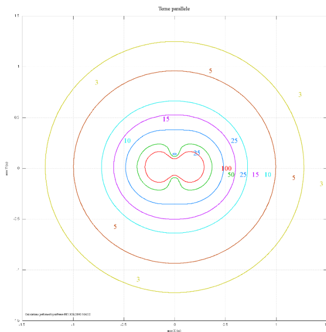
Figura 17: DPA tratto 6-5 (valori calcolati con l'ausilio del software Magic)
