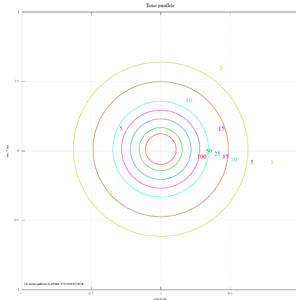
Figura 14: DPA tratto T09-7 (valori calcolati con l'ausilio del software Magic)
