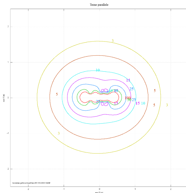
Figura 23: DPA tratto 3-2 (valori calcolati con l'ausilio del software Magic)
