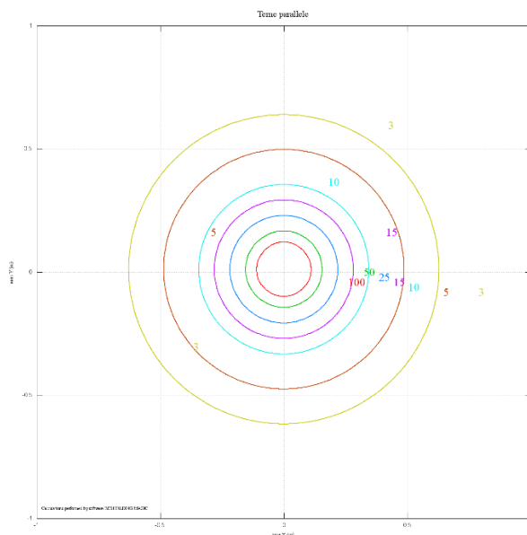
Figura 18: DPA tratto T05-5 (valori calcolati con l'ausilio del software Magic)
