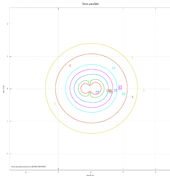
Figura 26: DPA tratto T01-1 (valori calcolati con l'ausilio del software Magic)
