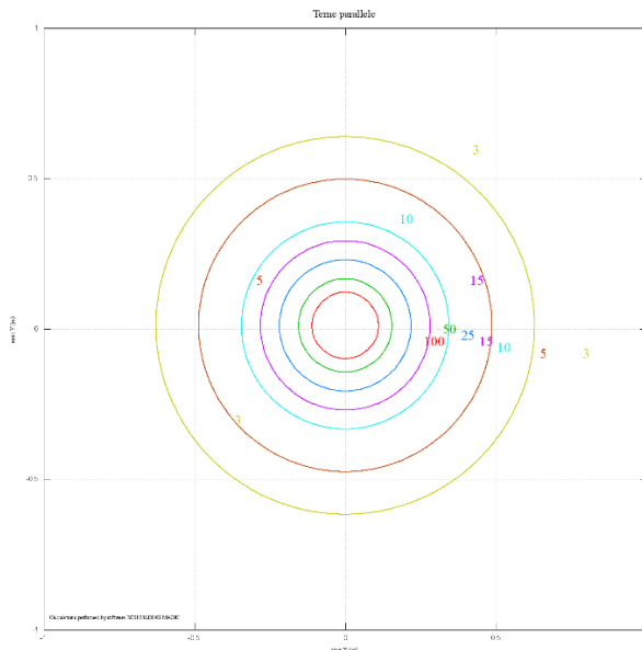
Figura 22: DPA tratto T03-3 (valori calcolati con l'ausilio del software Magic)
