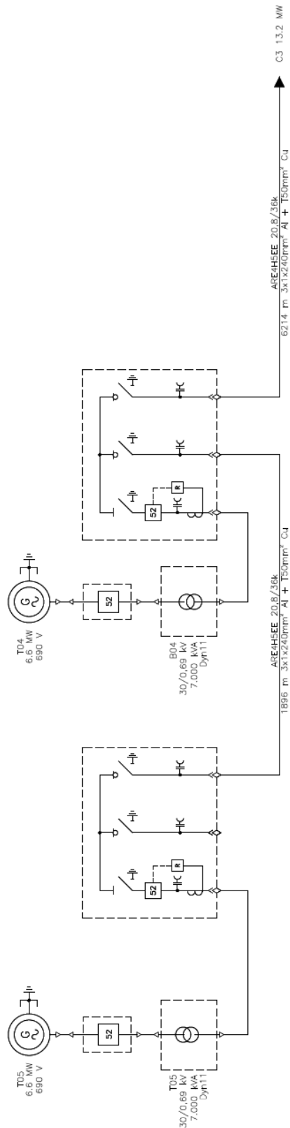
Figura 9: Schema collegamento Circuito 3
