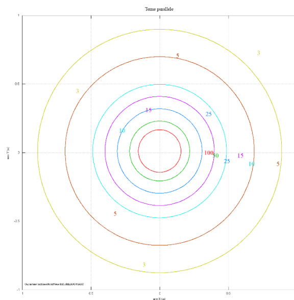
Figura 13: DPA tratto 8-7 (valori calcolati con l'ausilio del software Magic)
