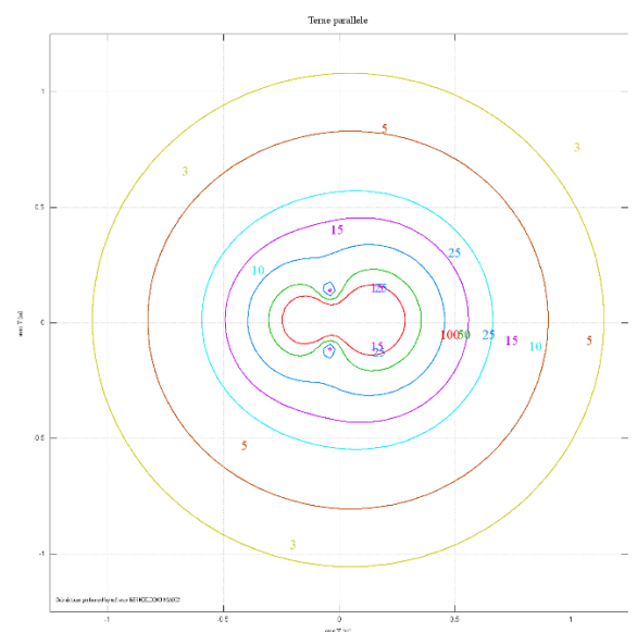
Figura 15: DPA tratto 7-6 (valori calcolati con l'ausilio del software Magic)
