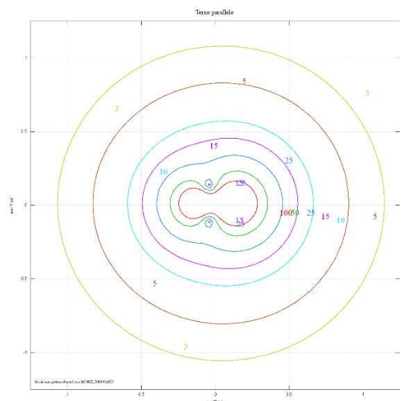
Figura 19: DPA tratto 5-4 (valori calcolati con l'ausilio del software Magic)
