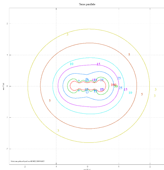
Figura 27: DPA tratto Esterno (valori calcolati con l'ausilio del software Magic)
