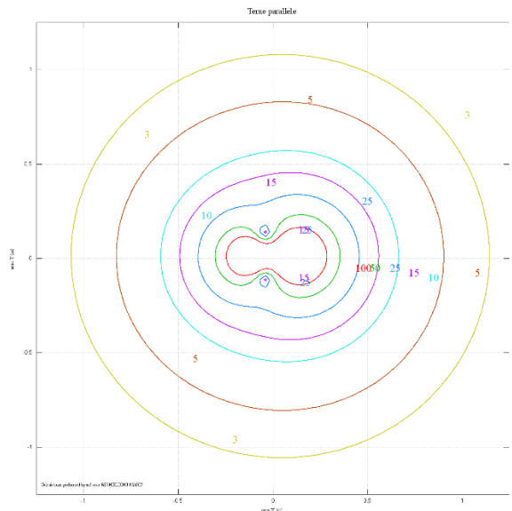
Figura 20: DPA tratto T04-4 (valori calcolati con l'ausilio del software Magic)
