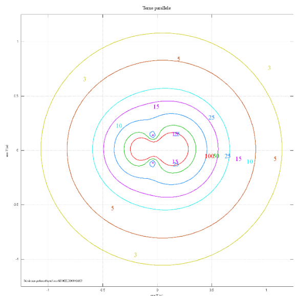
Figura 12: DPA tratto T07-8 (valori calcolati con l'ausilio del software Magic)
