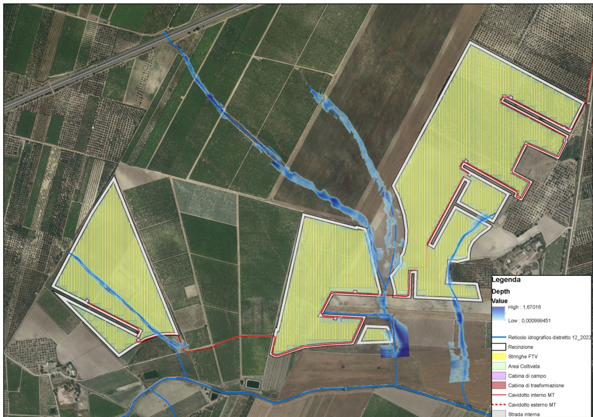
Figura 13: Tirante idrico
