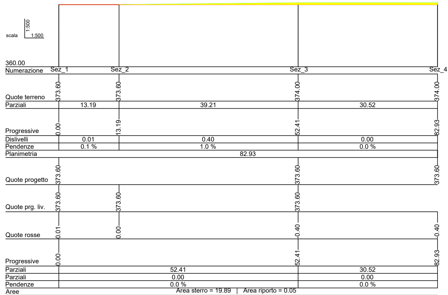
Profilo di Progetto ELE03
