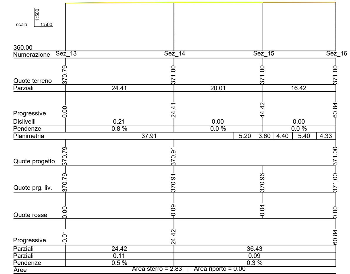
Profilo di Progetto_ELE06-TRATTO B
