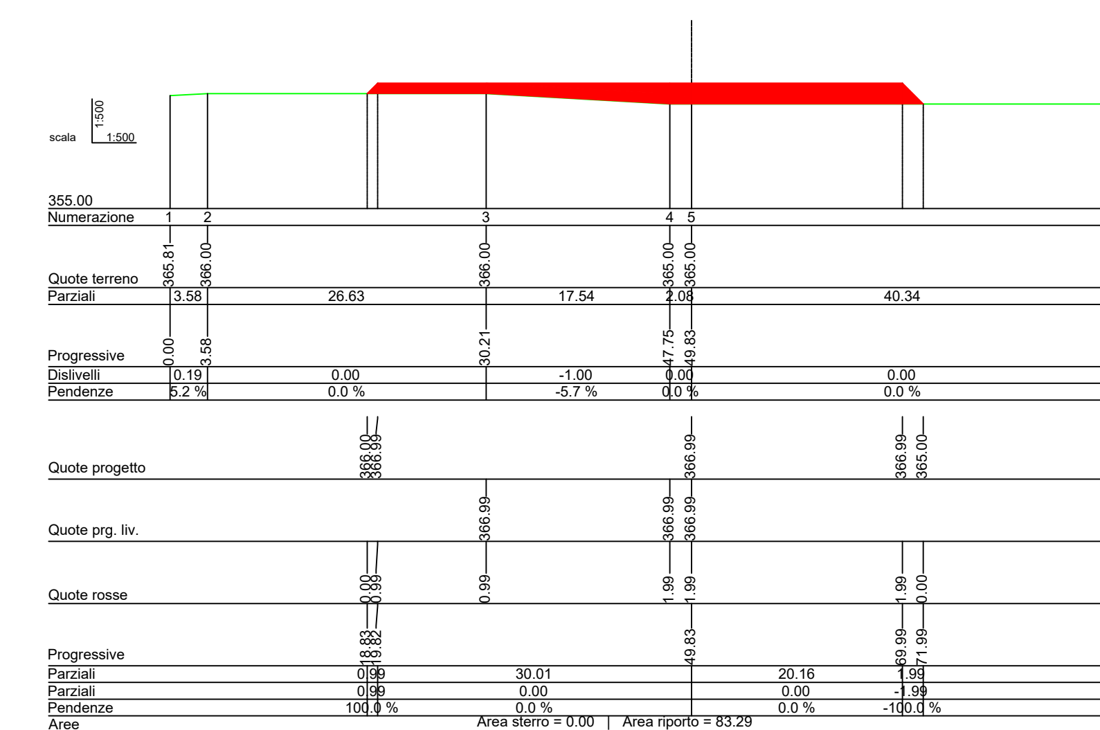
Sez_4 Prog.=83.139
