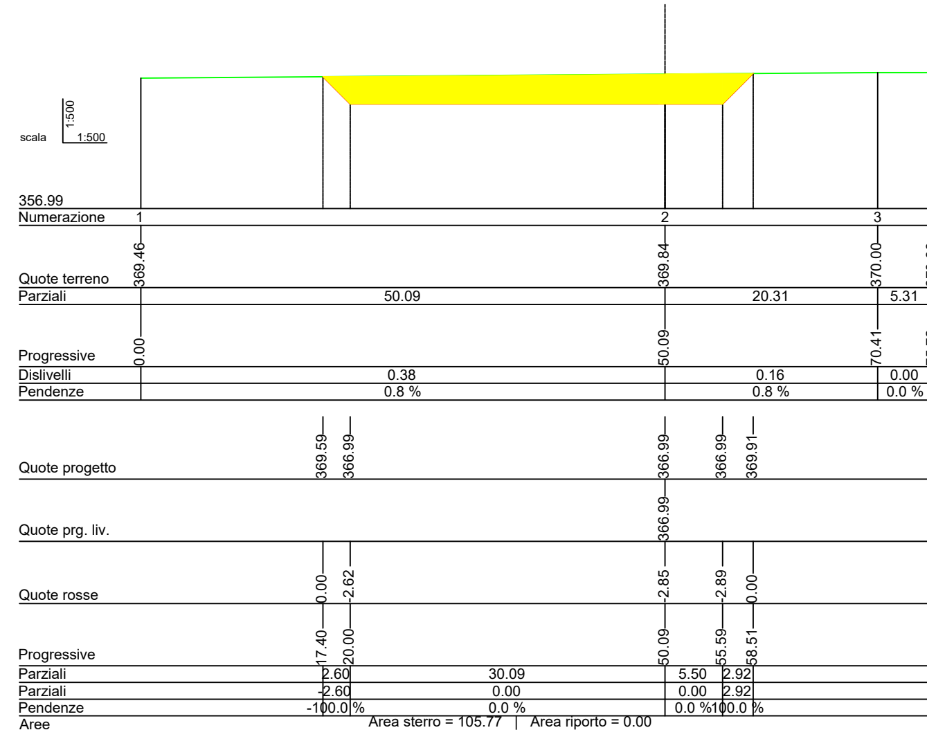
Sez_1 Prog.=0.000
