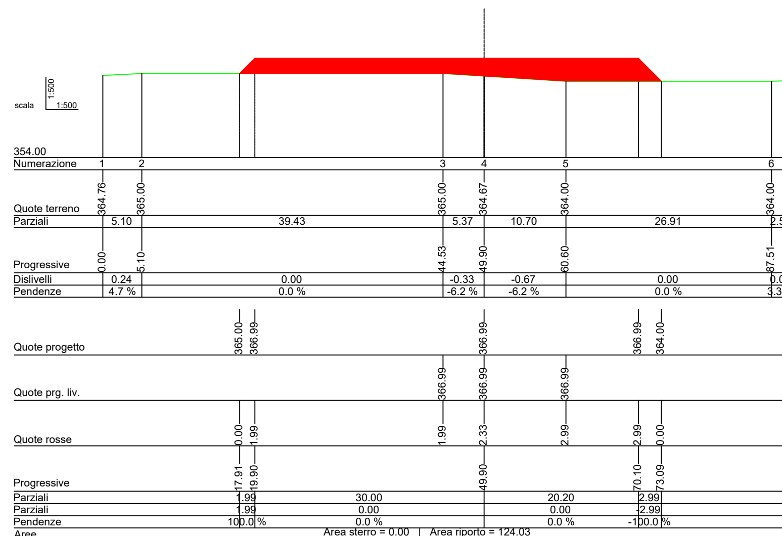
Sez_5 Prog.=96.670
