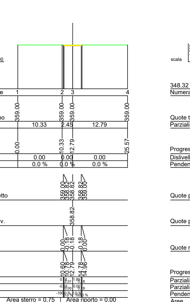
Sez_11 Prog.=216.648
