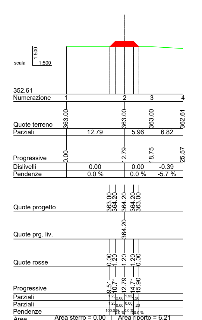
Sez_7 Prog.=136.670
