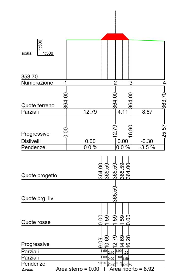
Sez_6 Prog.=116.670
