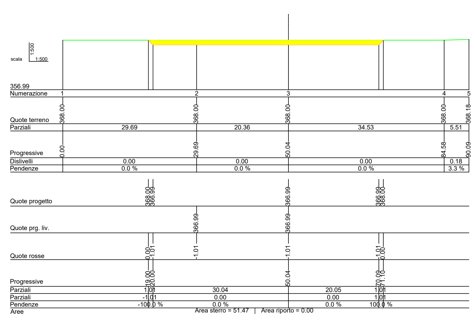
Sez_2 Prog.=25.414
