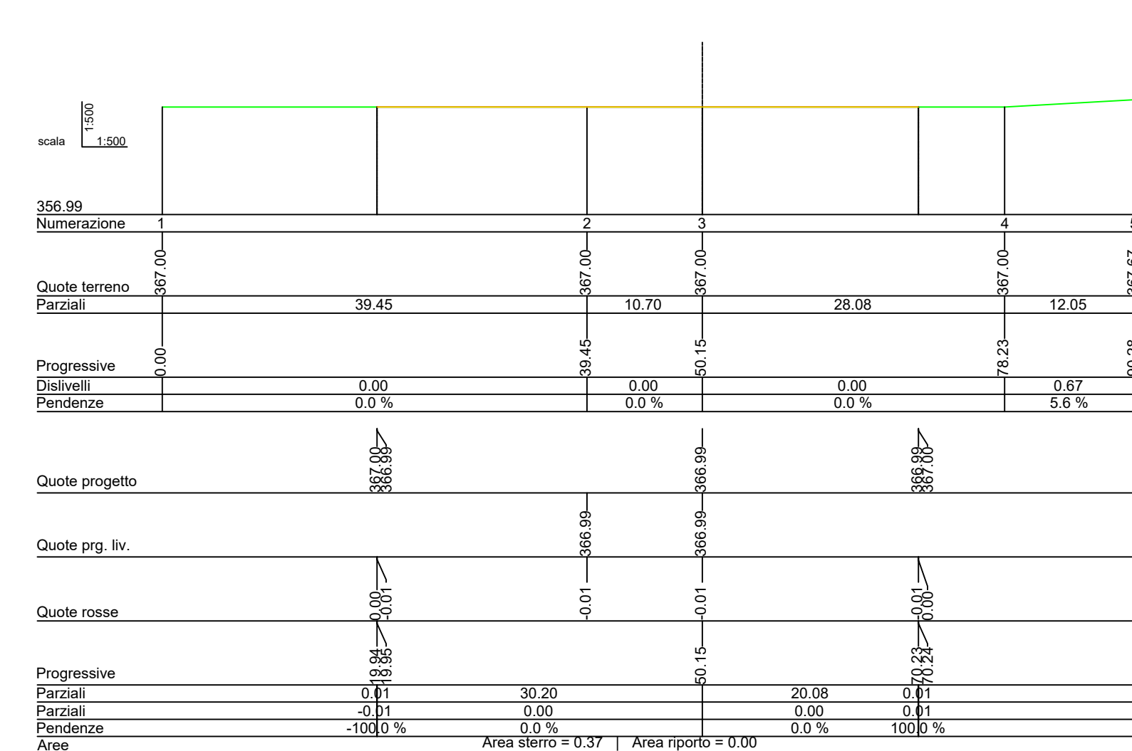
Sez_3 Prog.=48.697
