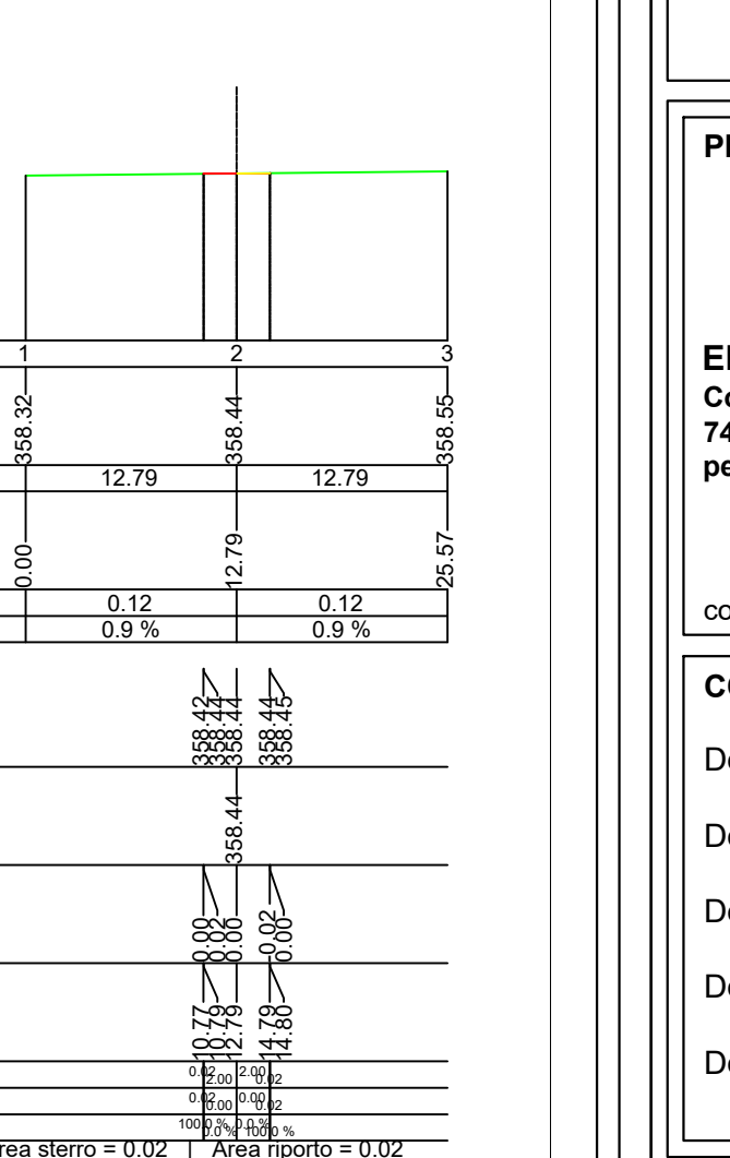
Sez_12 Prog.=223.160
