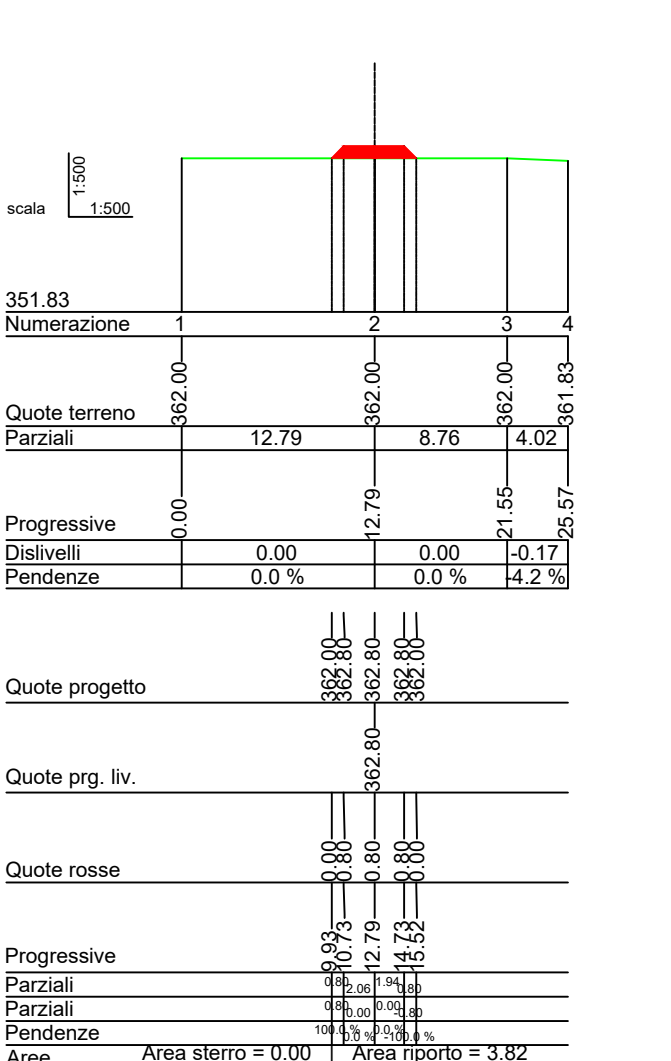
Sez_8 Prog.=156.670
