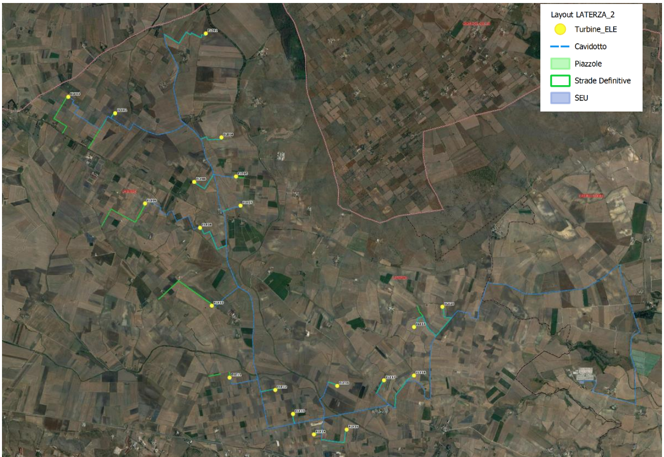
Figura 2.1-4: Area di intervento: layout di progetto su ortofoto
