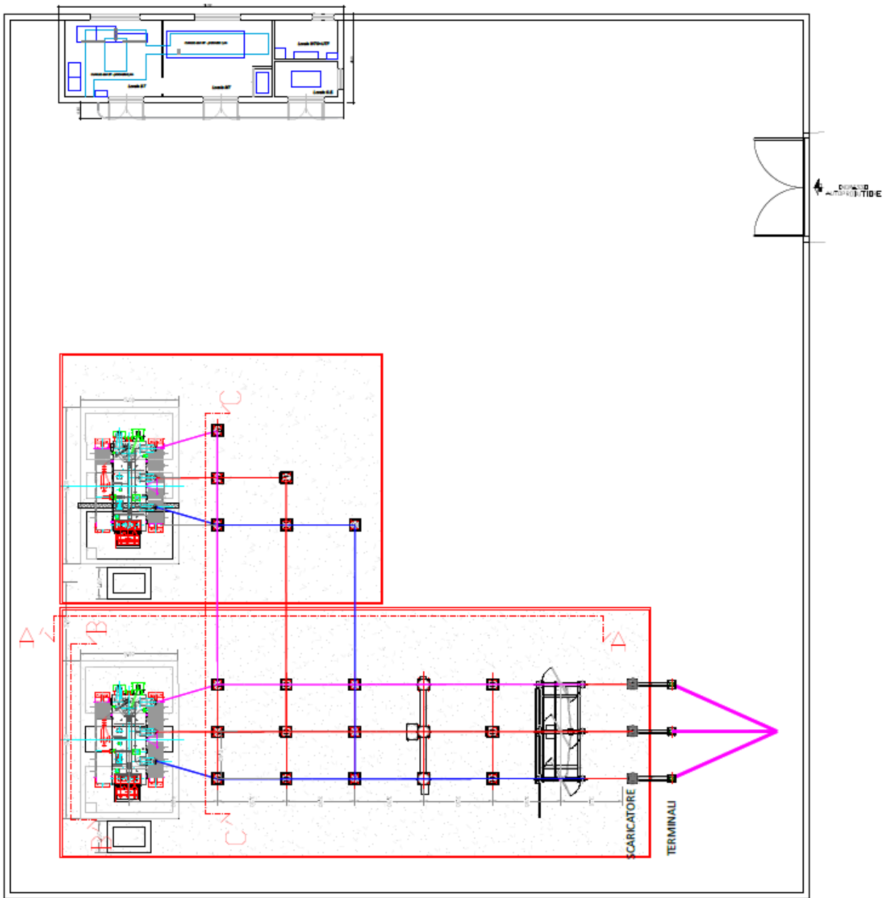
Figura 2.5-3: Stazione elettrica utente – schema planimetrico
