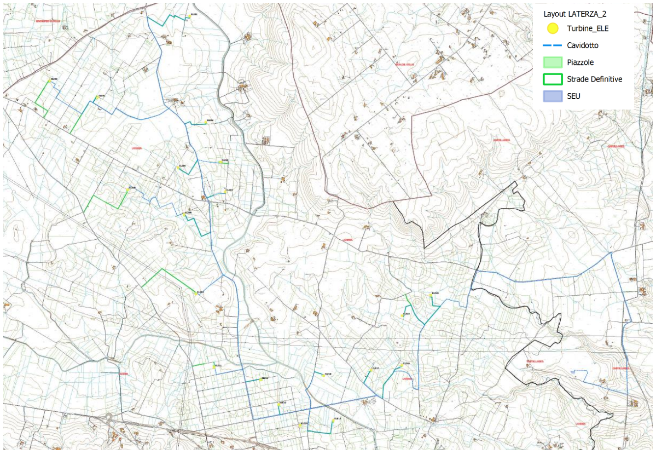
Figura 2.1-3: Layout del Parco Eolico su base CTR
