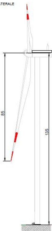
PROSPETTO LATERALE
