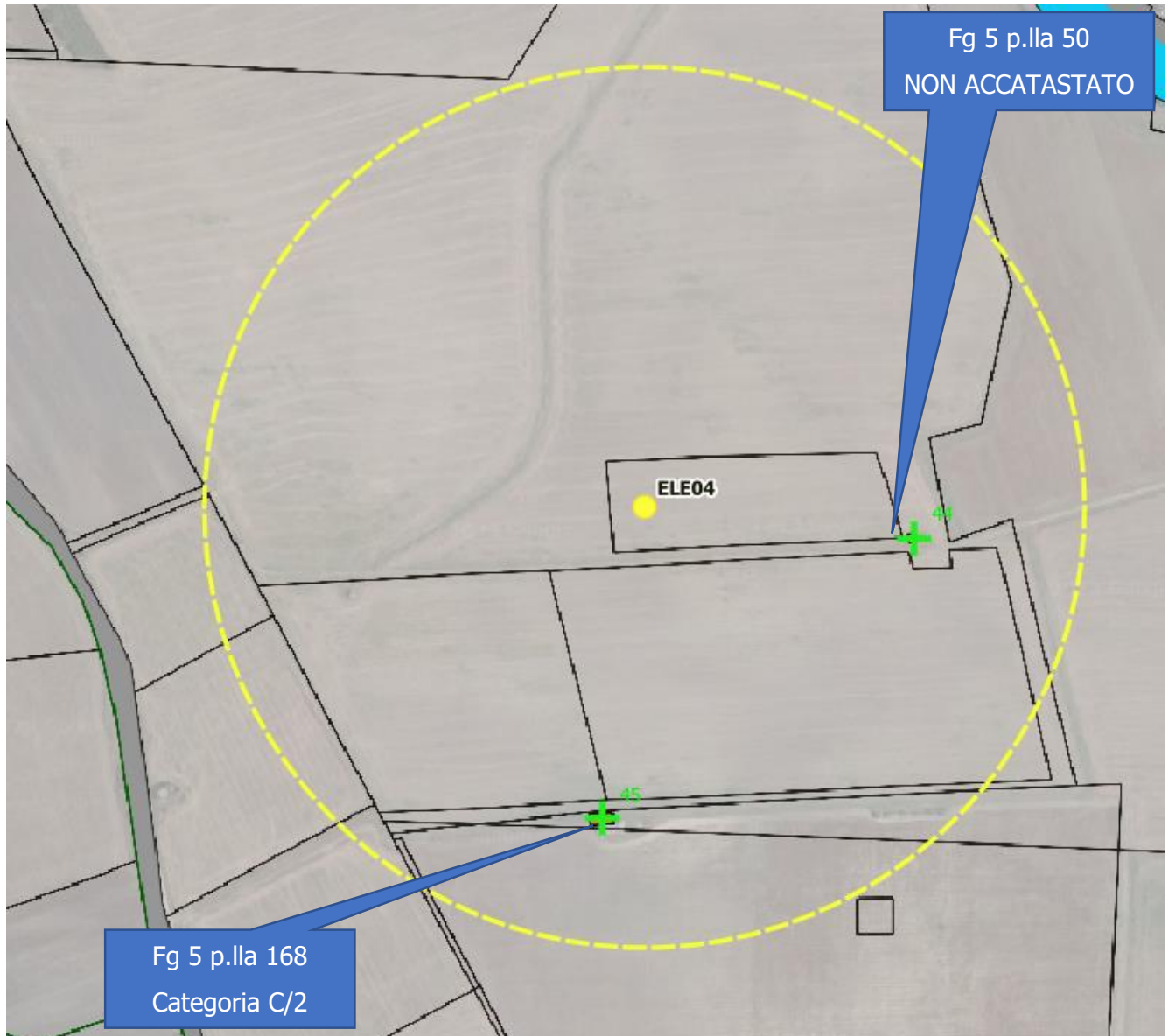
Figure 4 Particolare ELE04
