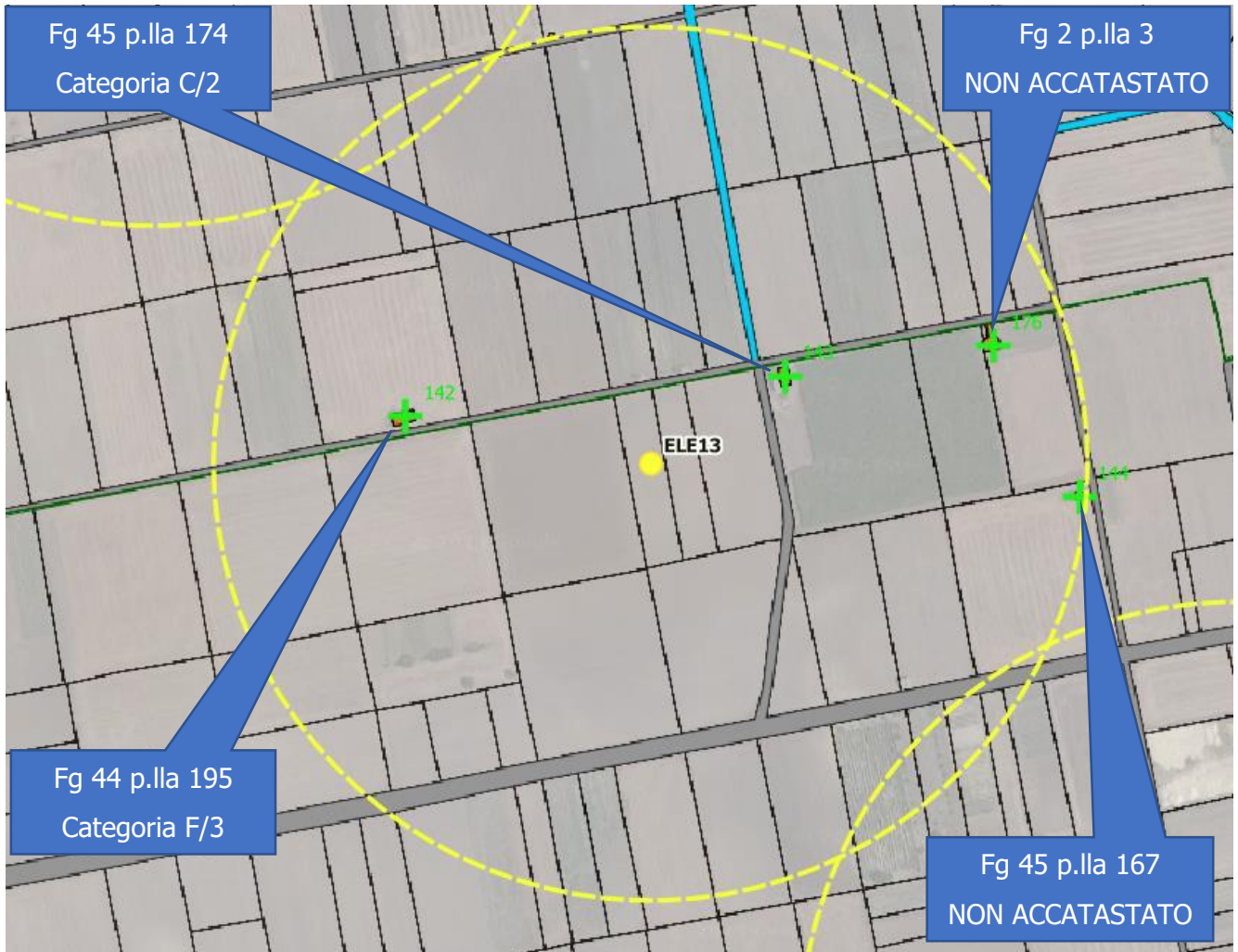
Figure 13 Particolare ELE13
