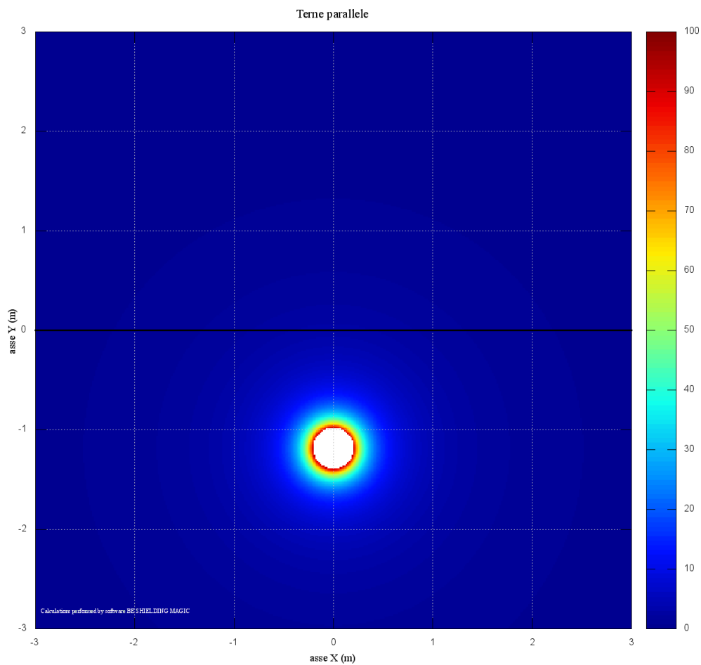
Figura 6: Anello PS, 1 terna, mappa 2D
