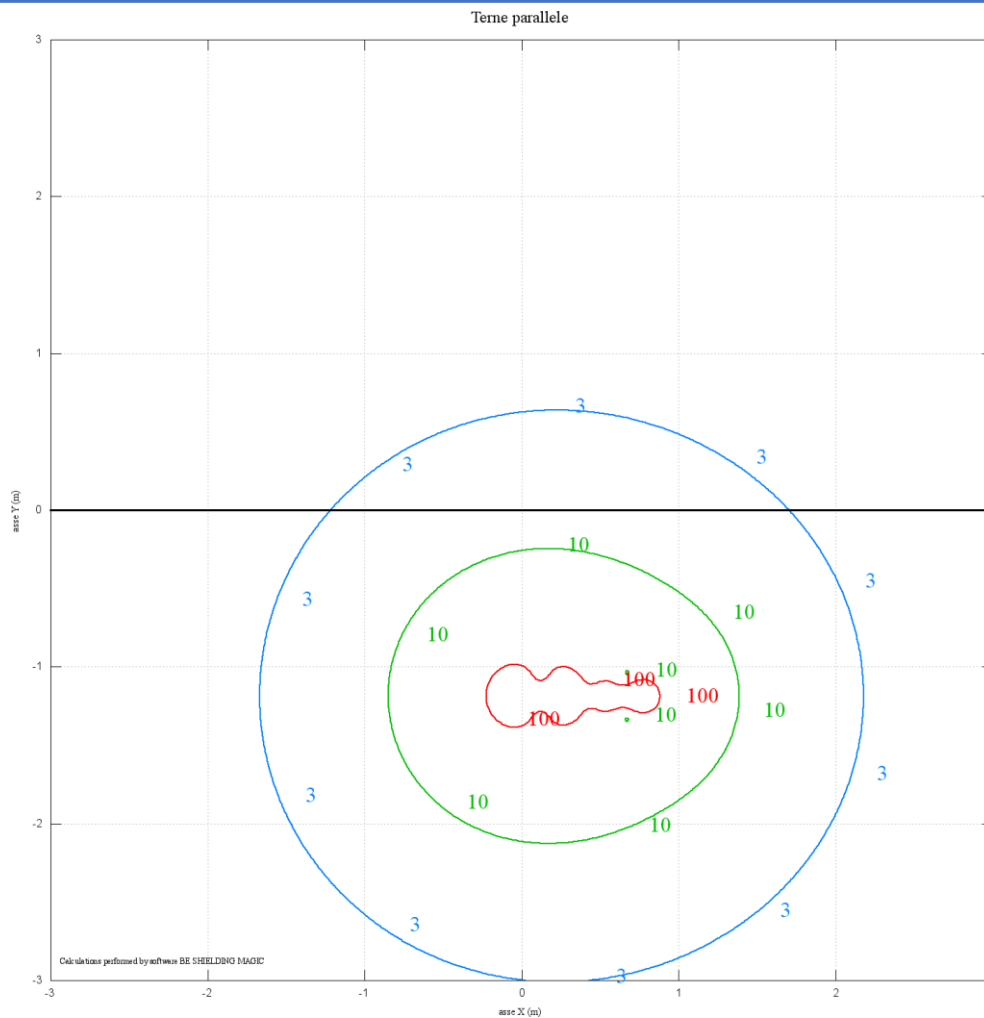
Figura 16: Anello PS e SPS, 4 terne, curve isolivello
