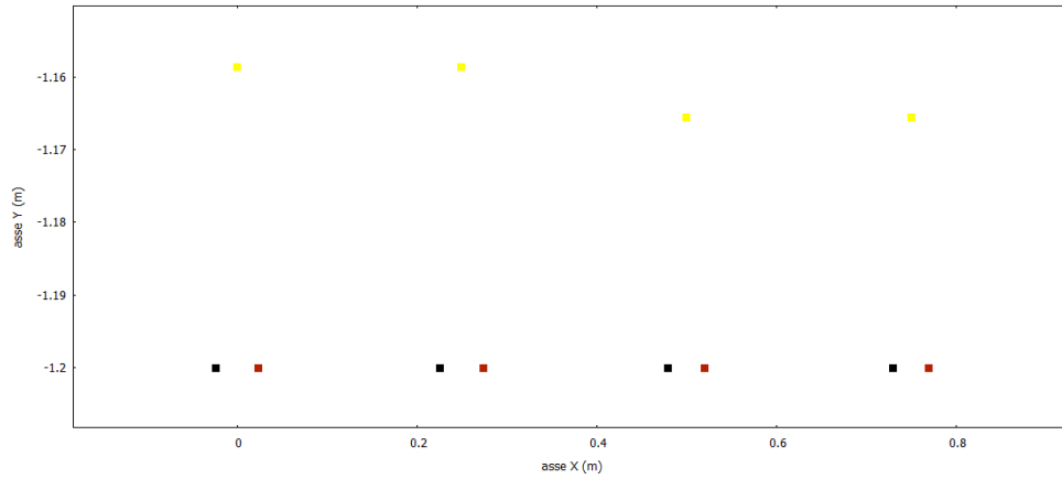
Figura 14: Anello PS e SPS, 4 terne, geometria
