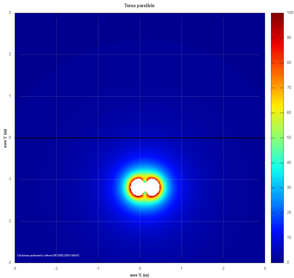
Figura 9: Anello PS, 2 terne, mappa 2D
