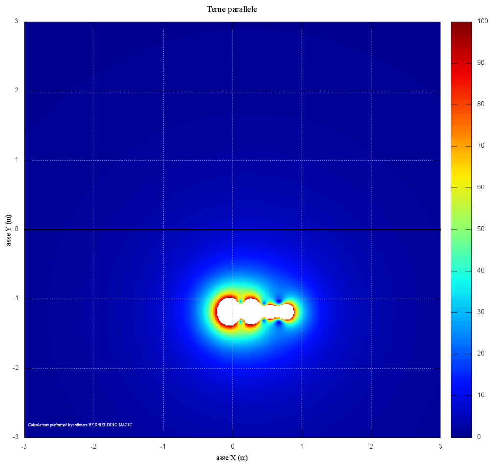
Figura 15: Anello PS e SPS, 4 terne, mappa 2D
