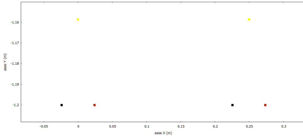
Figura 8: Anello PS, 2 terne, geometria
