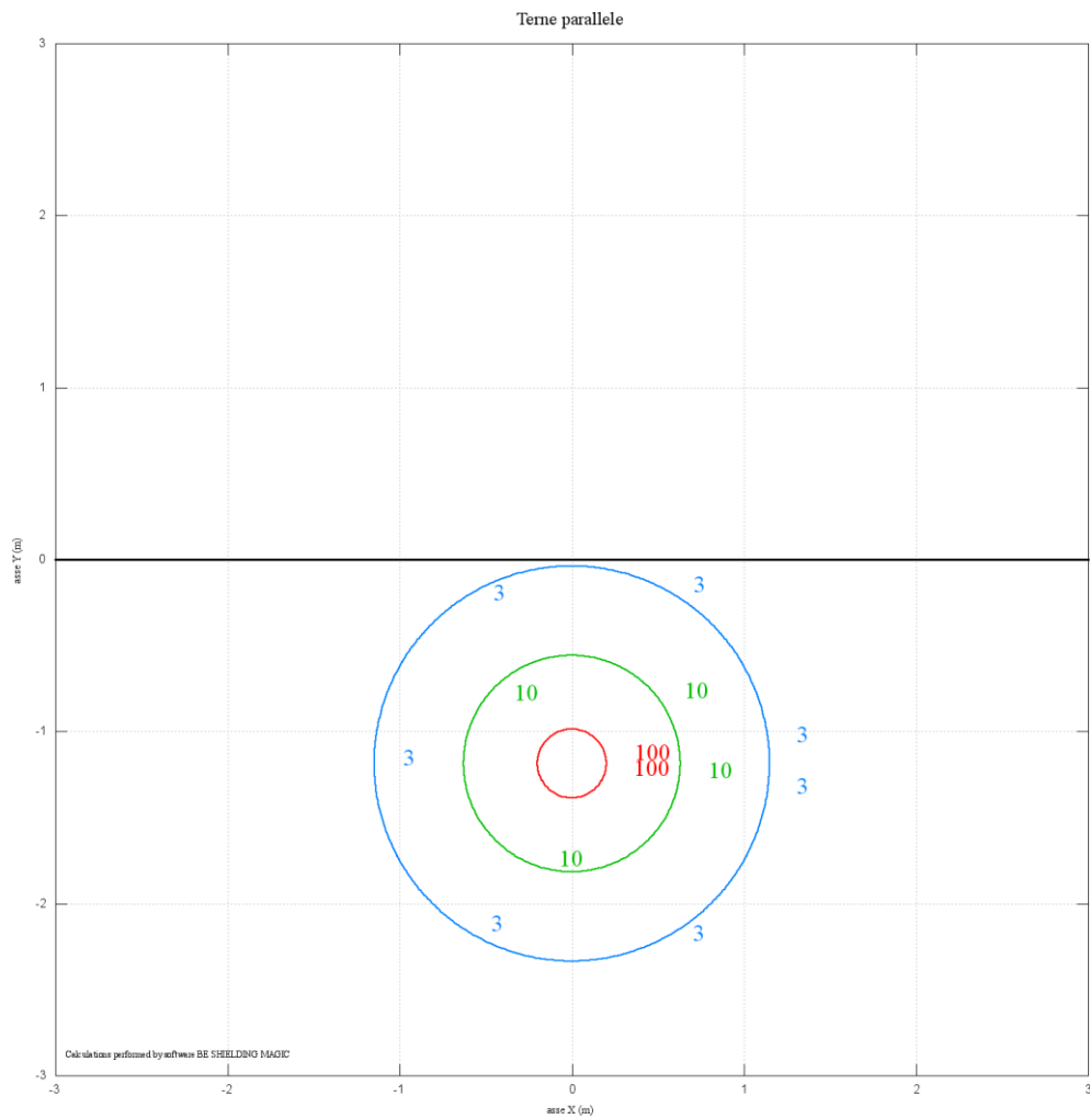
Figura 7: Anello PS, 1 terna, curve isolivello
