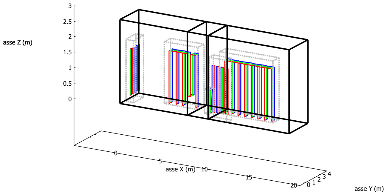
Figura 20: Cabina di Raccolta, geometria
