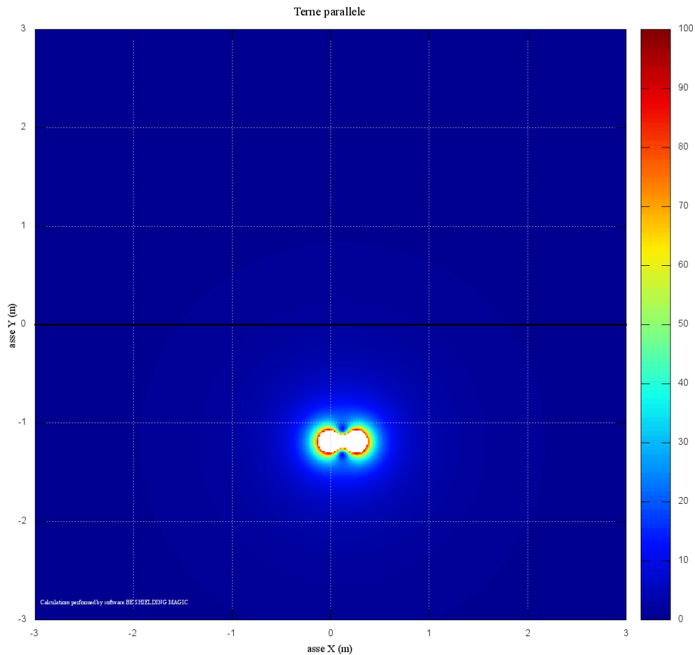
Figura 12: Anello SPS, 2 terne, mappa 2D
