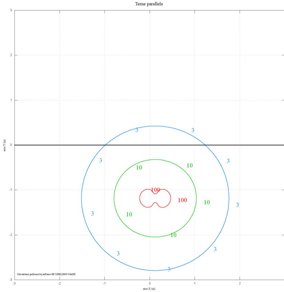
Figura 10: Anello PS, 2 terne, curve isolivello
