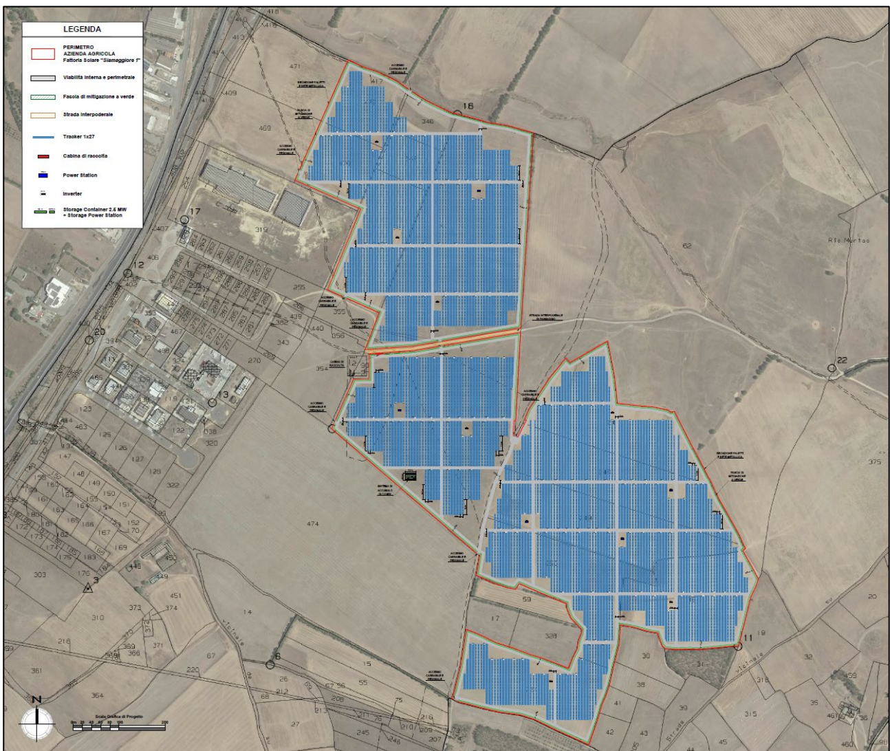
Figura 4: Layout di impianto su Catastale e Ortofoto. Riferimento Elaborato Grafico "2102_T.P.02_Layout Impianto su Orto-Catastale con viabilità interna_Rev00"
