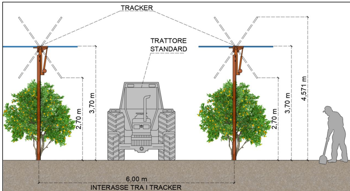
Figura 5: Esempio di impianto arboreo integrato con strutture fotovoltaiche
