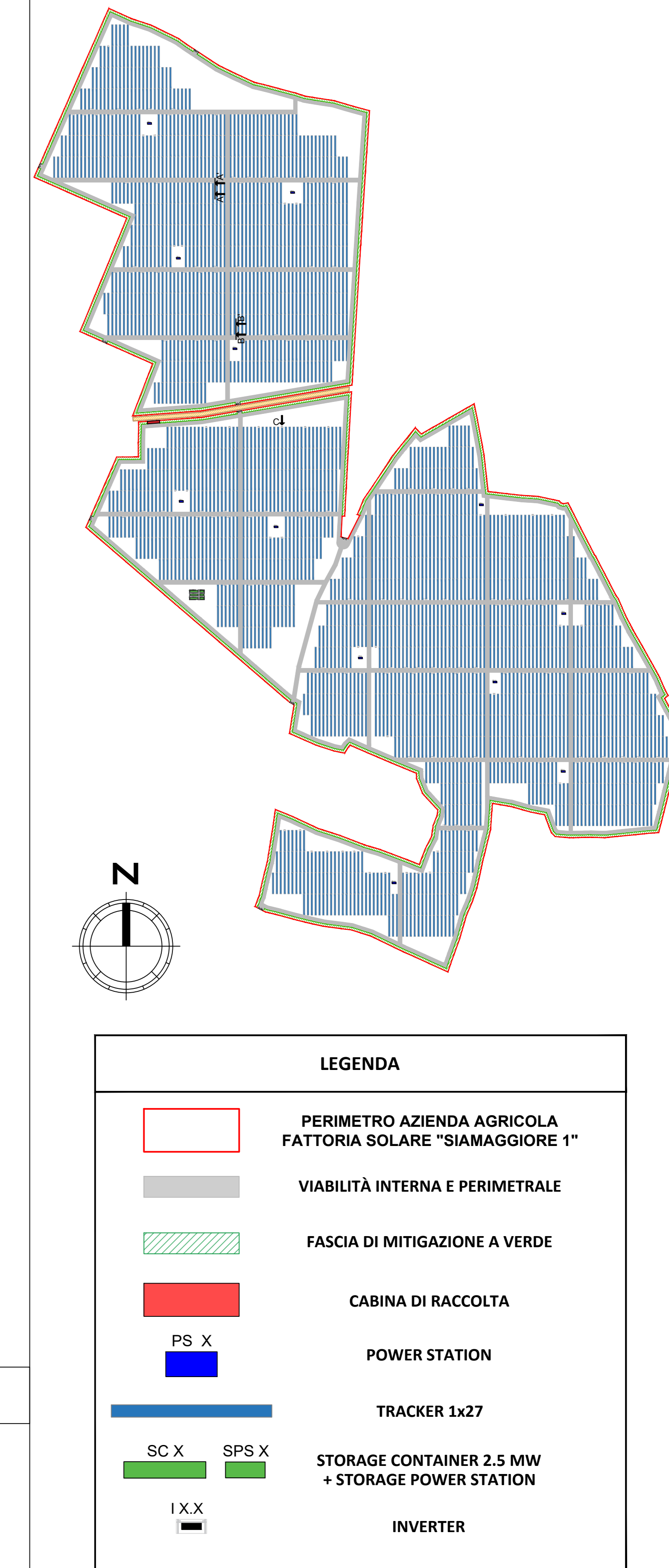
LAYOUT IMPIANTO - SCALA 1:5.000
