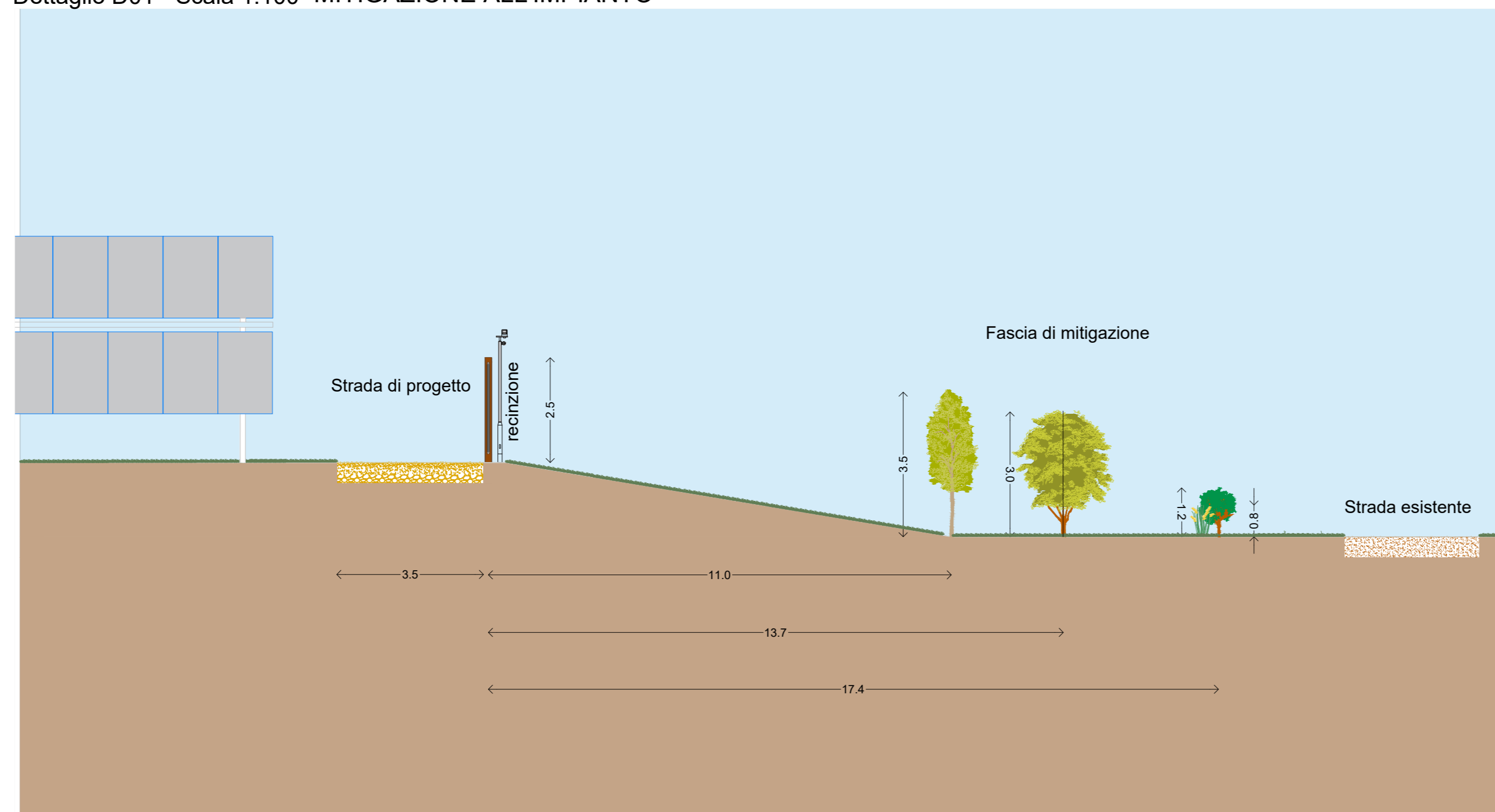
Dettaglio D01 - Scala 1:100 MITIGAZIONE TRASCORSI 10 ANNI
