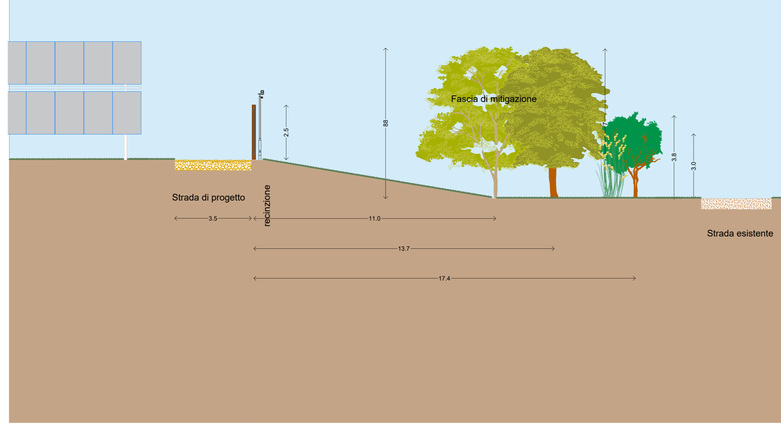
Dettaglio D02 - Scala 1:100 MITIGAZIONE ALL'IMPIANTO
