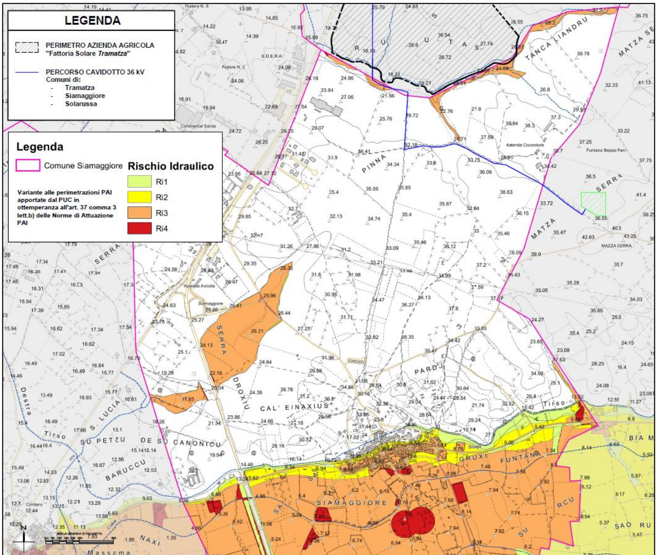
Figura 11: Variante alla perimetrazione PAI art. 37 comma 3 lett. b) PUC Siamaggiore – Carta rischio idraulico Riferimento Elaborato Grafico "2104_T.A.09b_Cartografia PUC - Variante Perimetrazioni PAI - Rischio Idraulico_Rev00"
