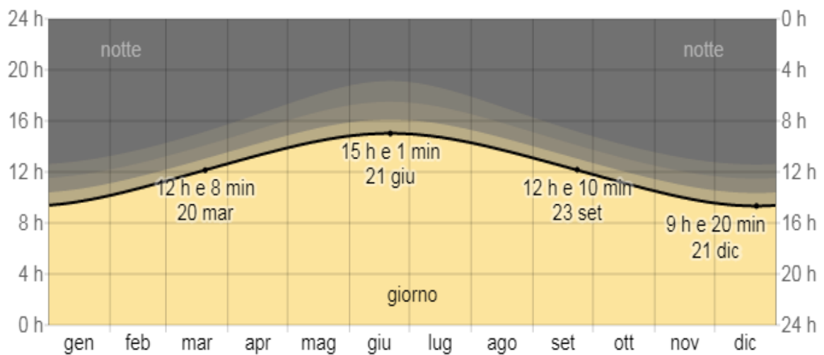
Figura 16: Variazioni crepuscolari
