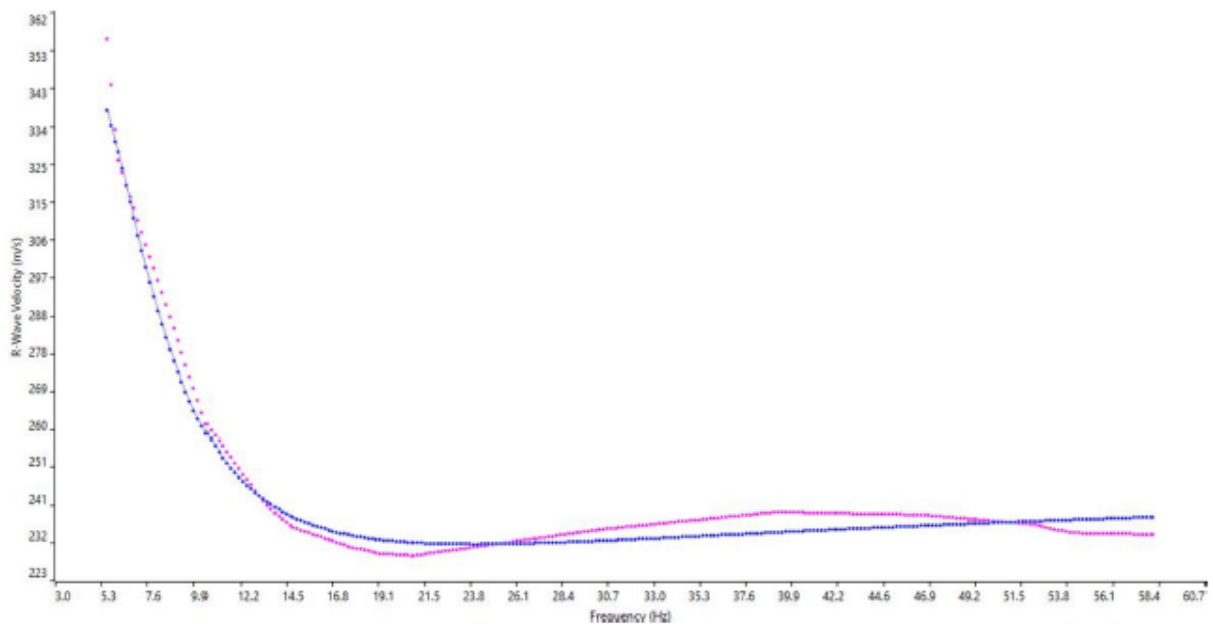
Figura 16: Curva sperimentale (in rosa) e teorica (in blu)
