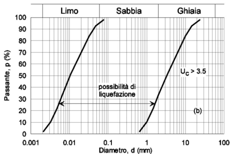
Figura 19: Fusi granulometrici dei terreni soggetti a liquefazione
