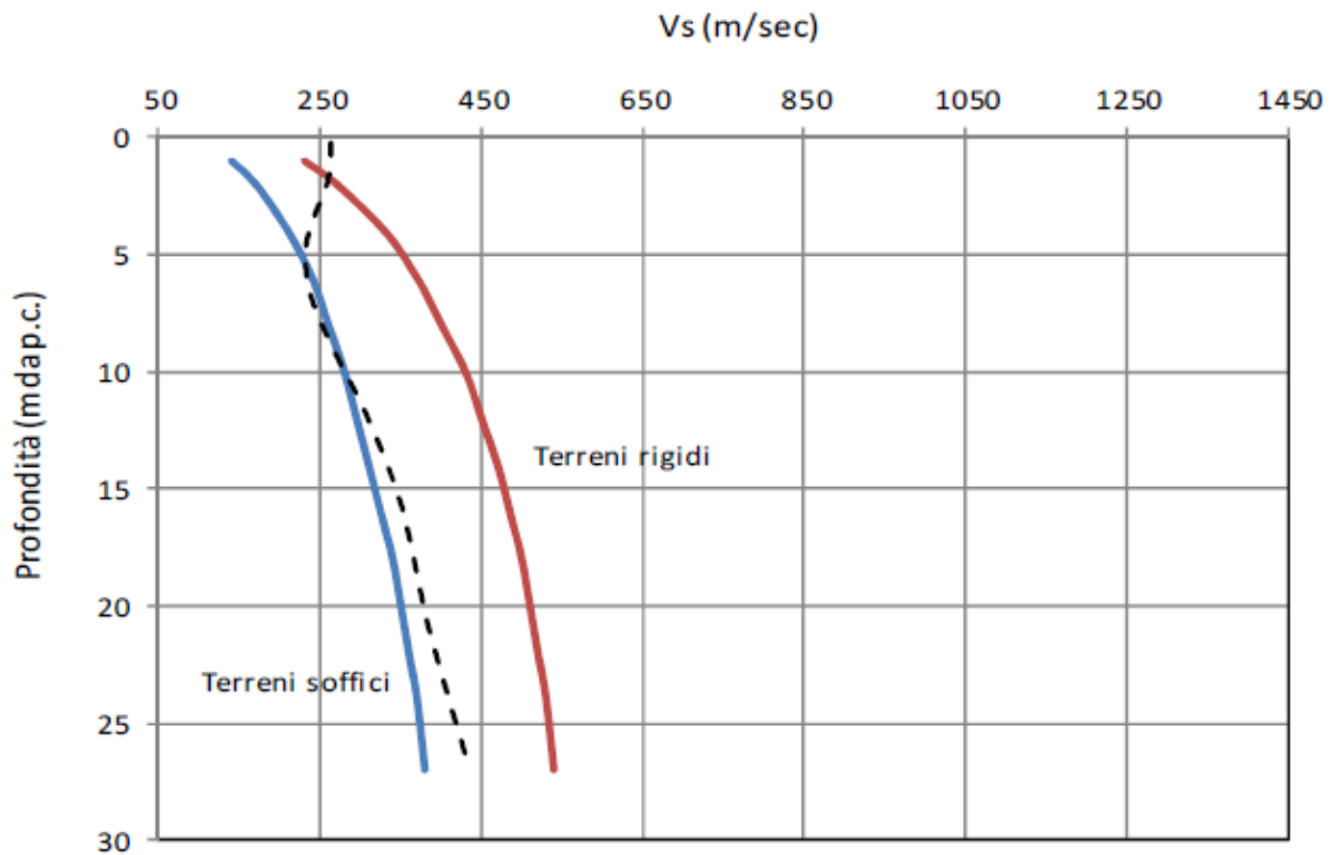
Figura 18: Classificazione dei terreni secondo le NTC 2018
