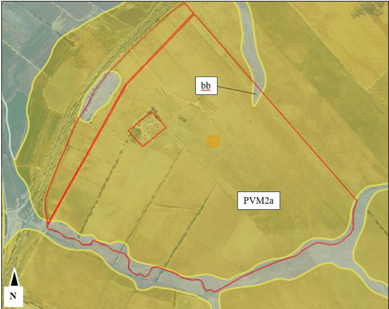
Figura 6: Stralcio della carta geologica dell'area (Fonte PPR)
