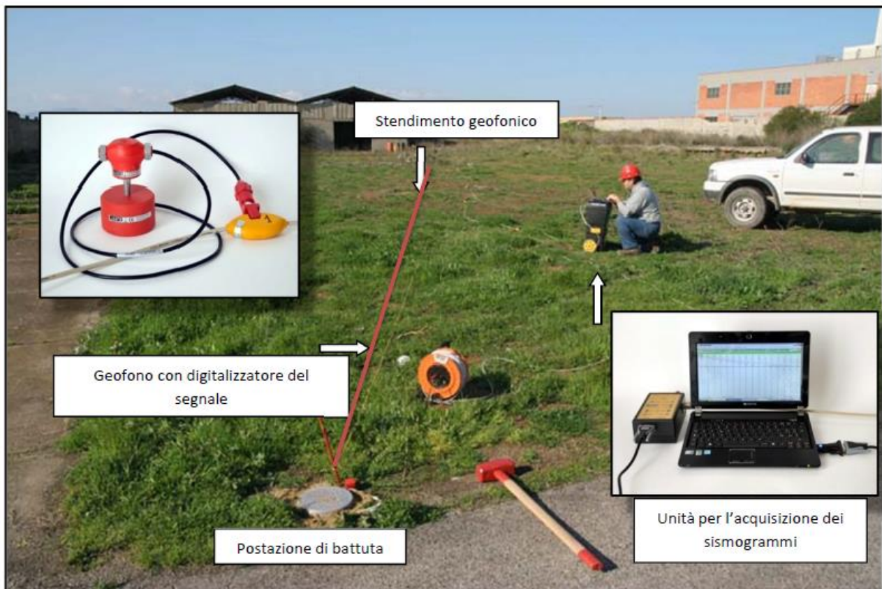
Figura 13: Configurazione dello strumento di misura
