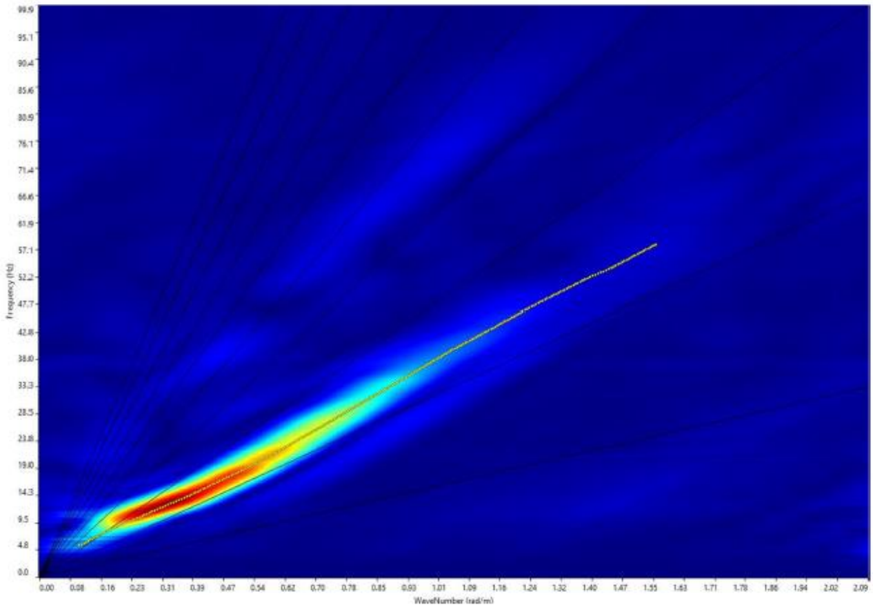
Figura 15: Spettro
