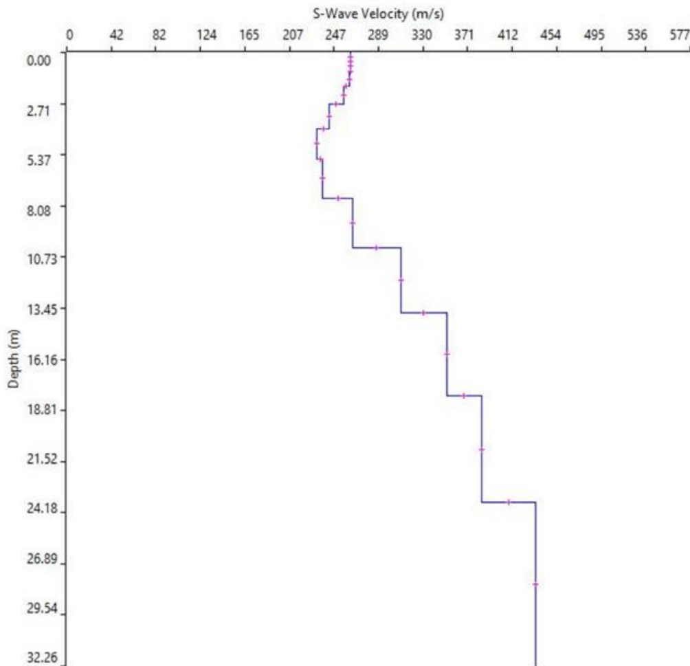
Figura 17: Profilo monodimensionale Vs – profondità
