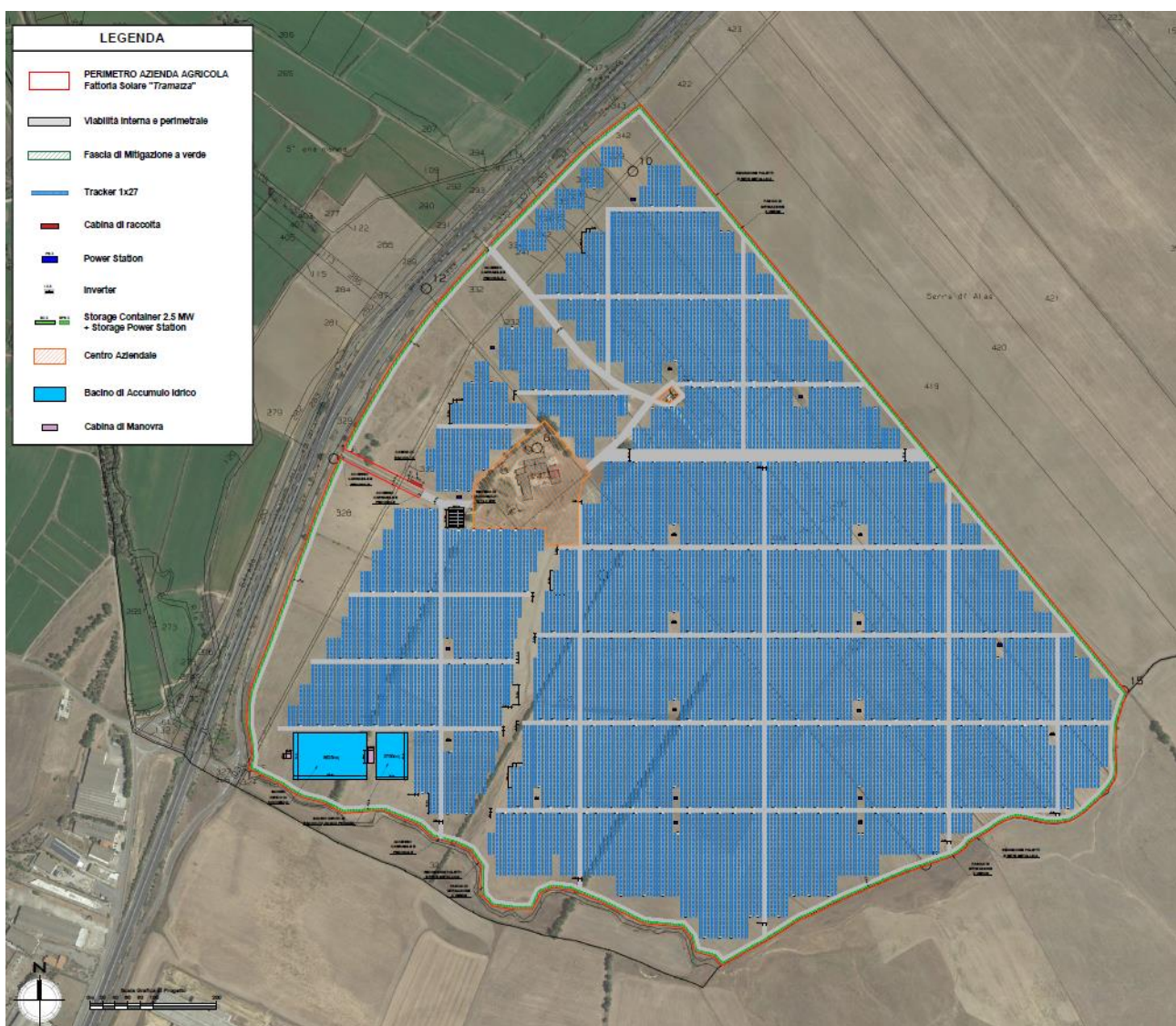
Figura 4: Layout di impianto su Catastale e Ortofoto. Riferimento Elaborato Grafico "2104_T.P.02_Layout Impianto su Orto-Catastale con viabilità interna_Rev00"
