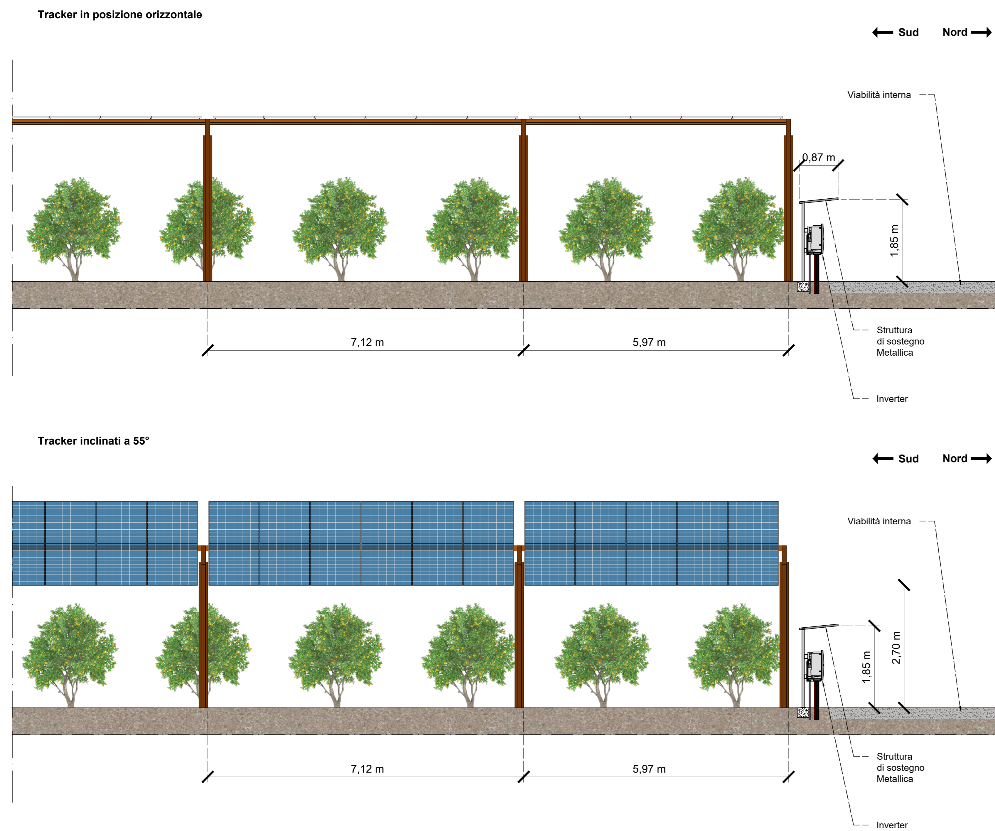
DETTAGLIO POSIZIONAMENTO INVERTER (VISTA C) - SCALA 1:20
