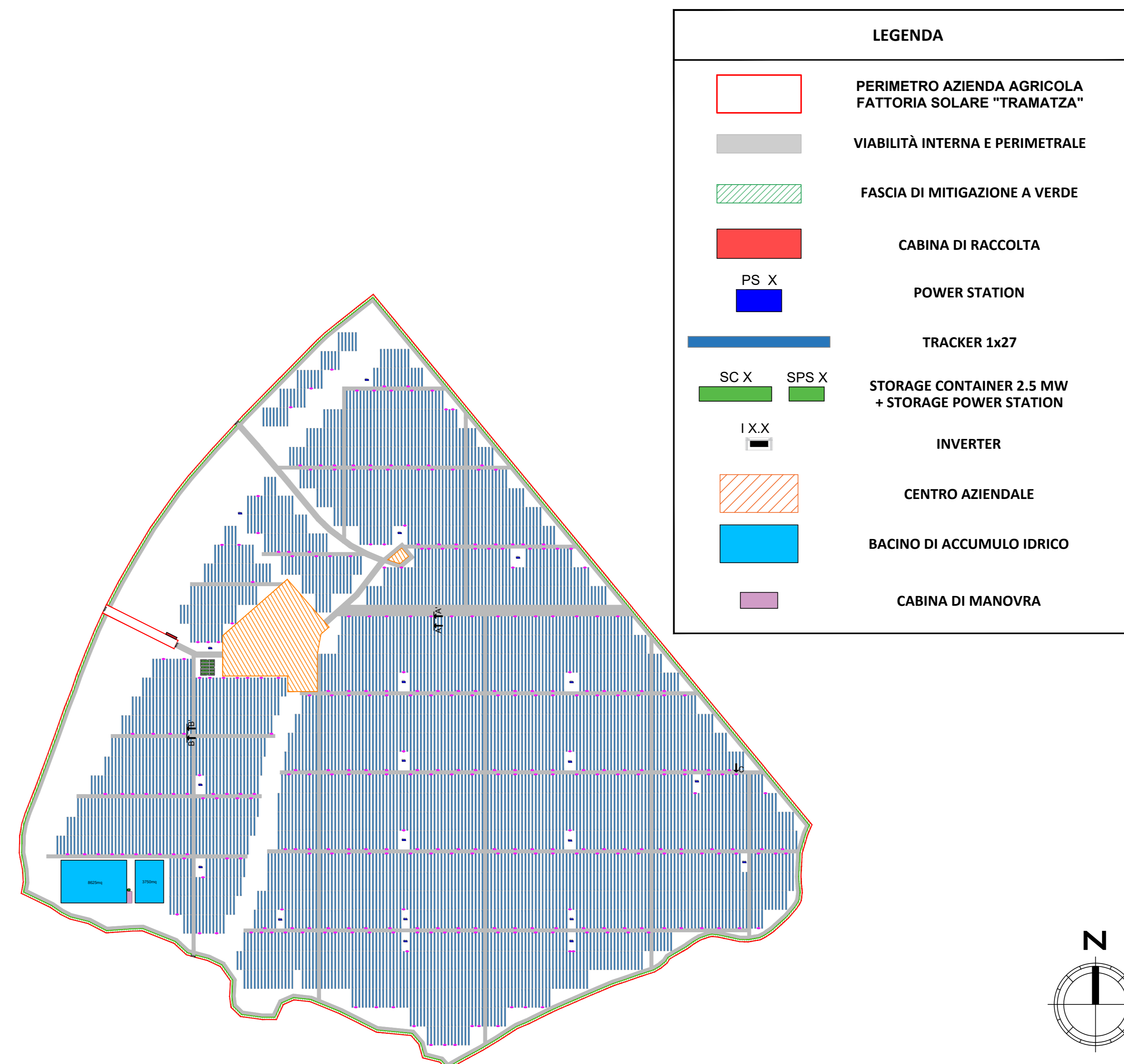
LAYOUT IMPIANTO - SCALA 1:5.000
