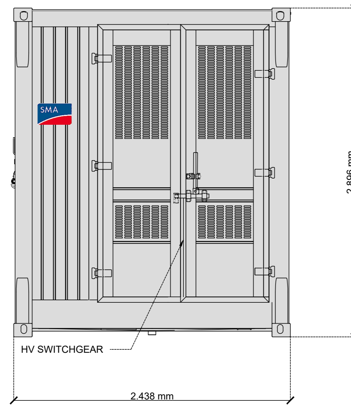
PROSPETTO FRONTALE SPS - SCALA 1:20
