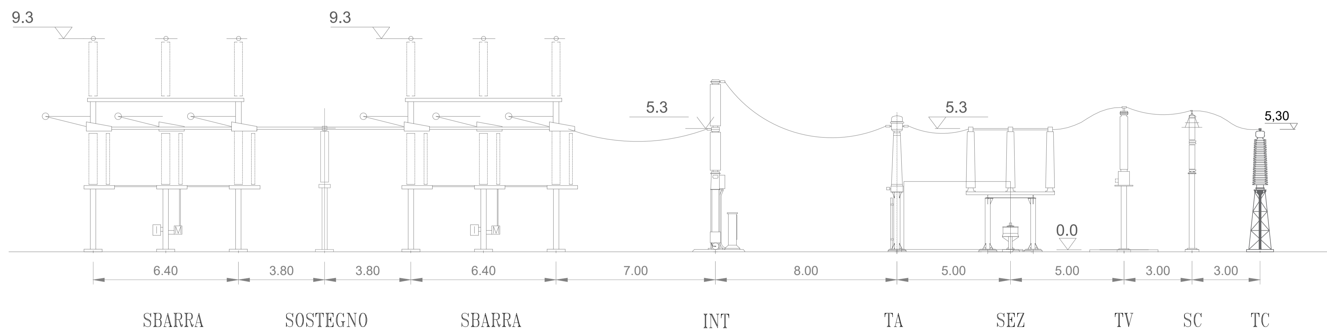
Sezione stallo linea cavo 220kV
