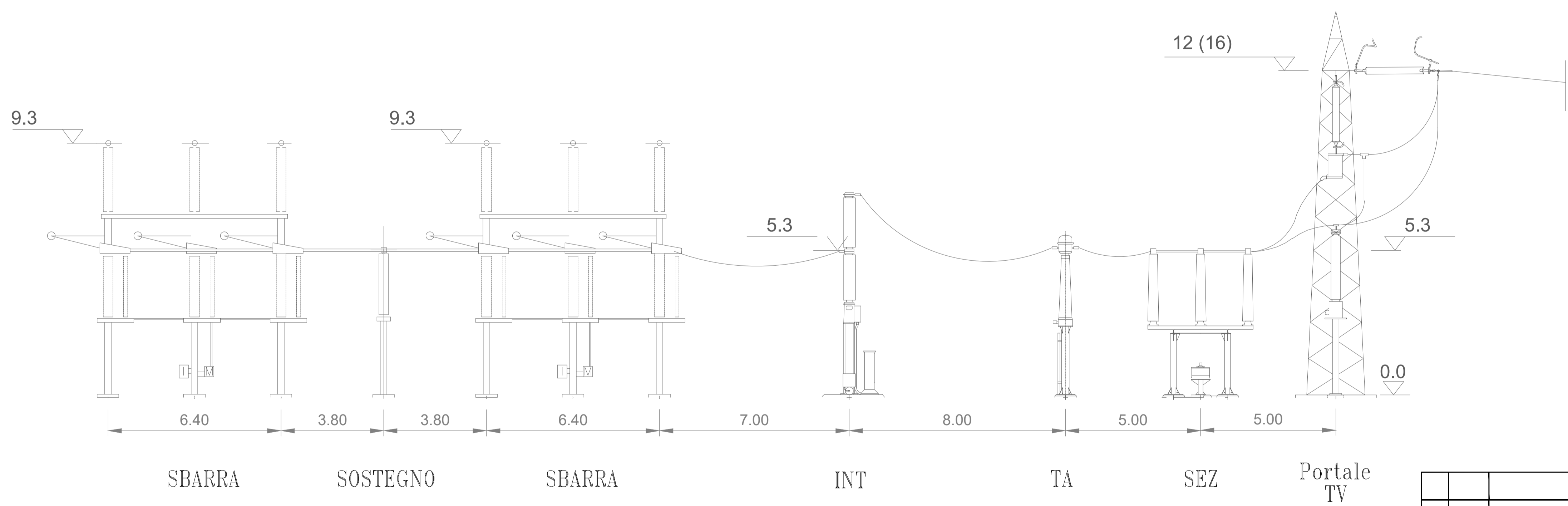
Sezione stallo linea aerea 220kV
