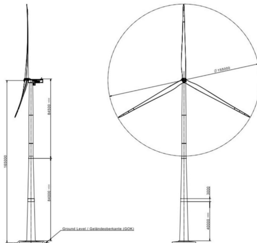
Figura 8 - SG 6.0-170 135 m
