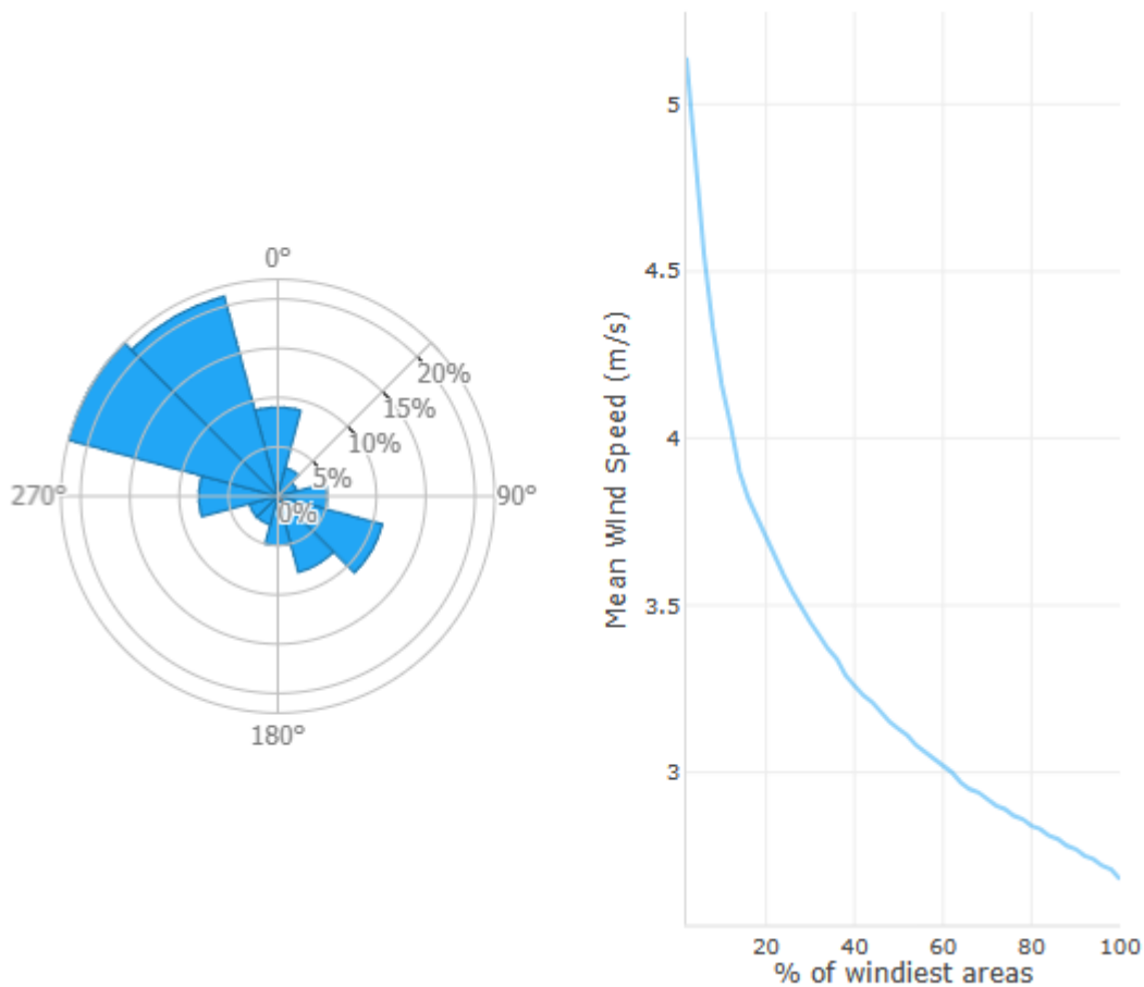
Figura 36: Wind Speed Rose a 10 m relativa all'area di impianto. La velocità del vento a 10 m risulta pari a 4.16 m/s
