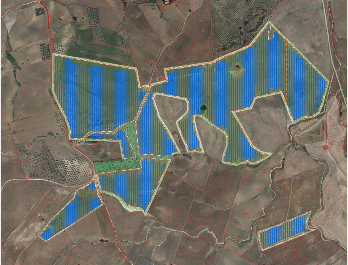
Figura 48: Layout definitivo e aree di mitigazione e/o compensazione
