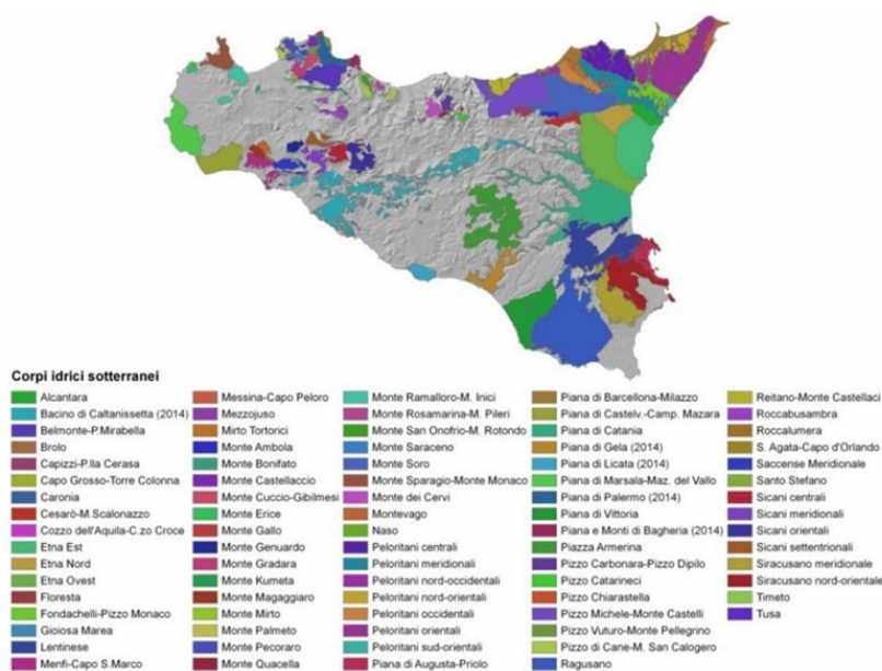
Figura 16: Corpi idrici sotterranei della Regione Sicilia (Fonte: Arpa Sicilia)
