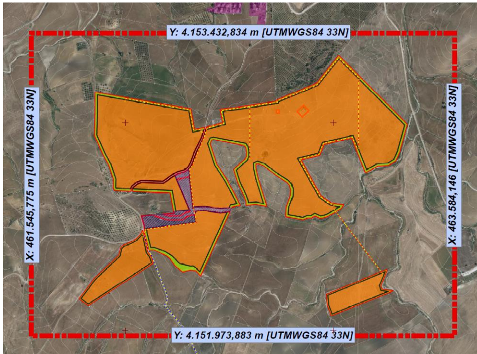
Figura 2: coordinate geografiche del perimetro racchiudente l'area di progetto fornite nel sistema di riferimento UTM WGS84 - stralcio dell'elaborato grafico "TAVA12a16 - Carta con localizzazione georeferenziata")
