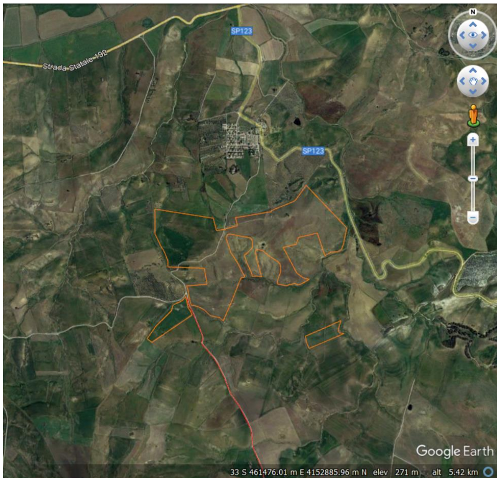
Figura 3: Accesso all'area del parco agrivoltaico da circa 40 MWp sito nel Comune di Ramacca (CT) - Fonte: Google Earth
