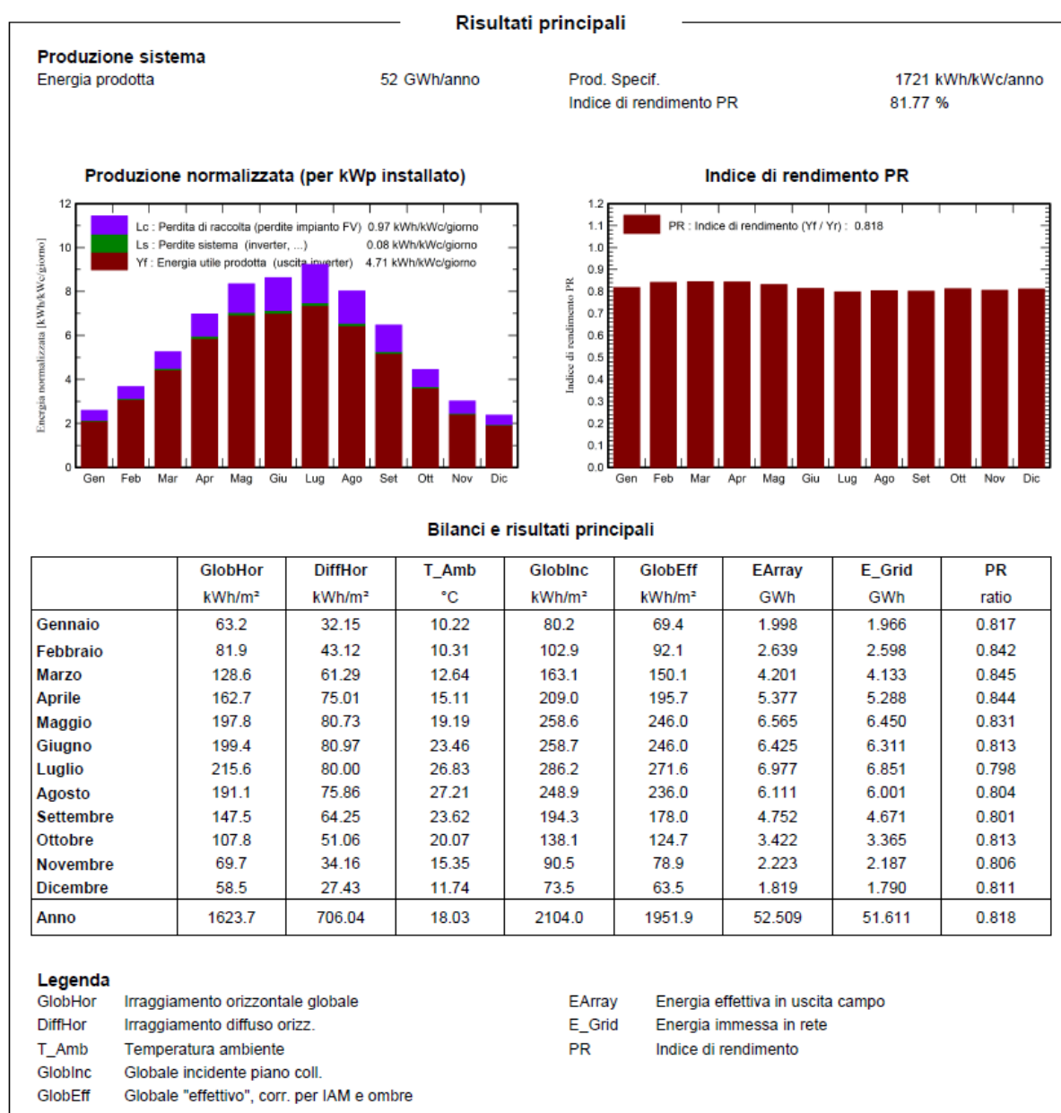
Figura 4: Risultati ottenuti con PVSyst
