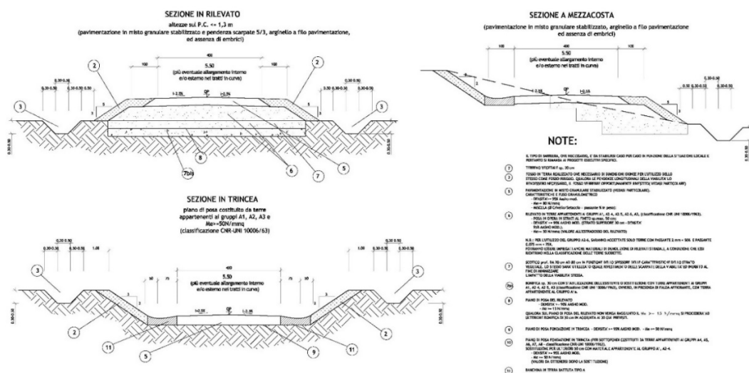
Figura 31: dettagli relativi alle caratteristiche costruttive della viabilità interna al parco
