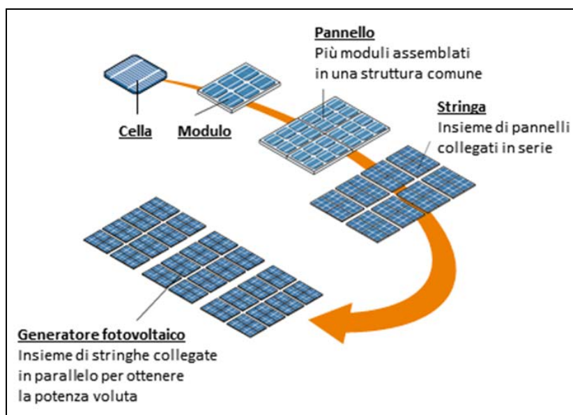
Figura 32: unità elementari del generatore fotovoltaico
