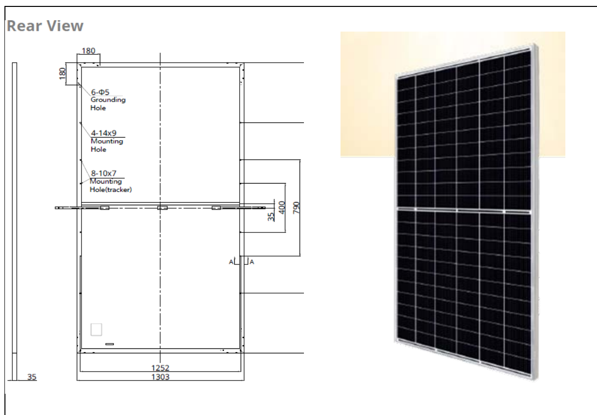
Figura 33: pannello FV fino a 665 Wp con dimensioni 2384 x 1303 x 35 mm
