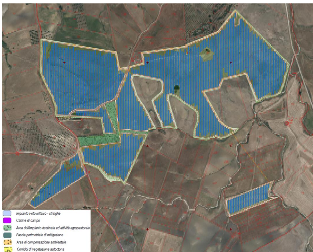
Figura 2: layout definitivo su cartografia catastale e ortofoto
