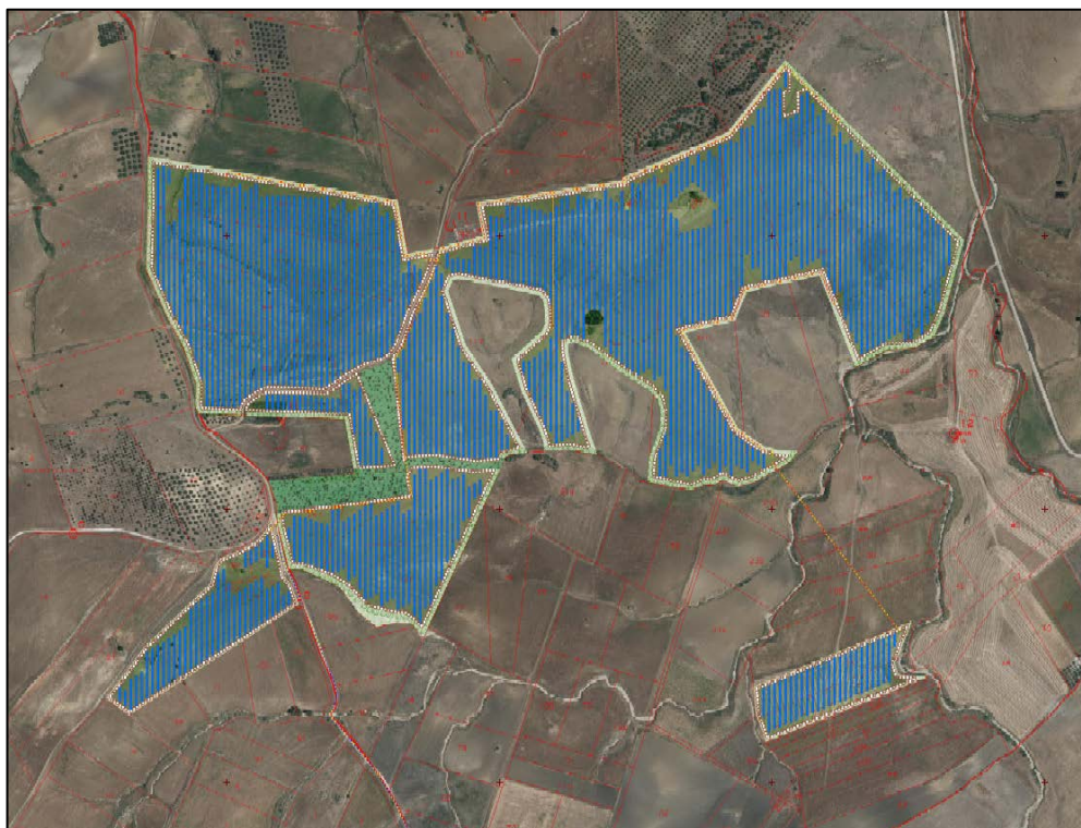
Figura 6: stralcio dell'elaborato grafico "A12A17 - Layout definitivo su cartografia catastale e ortofoto "
