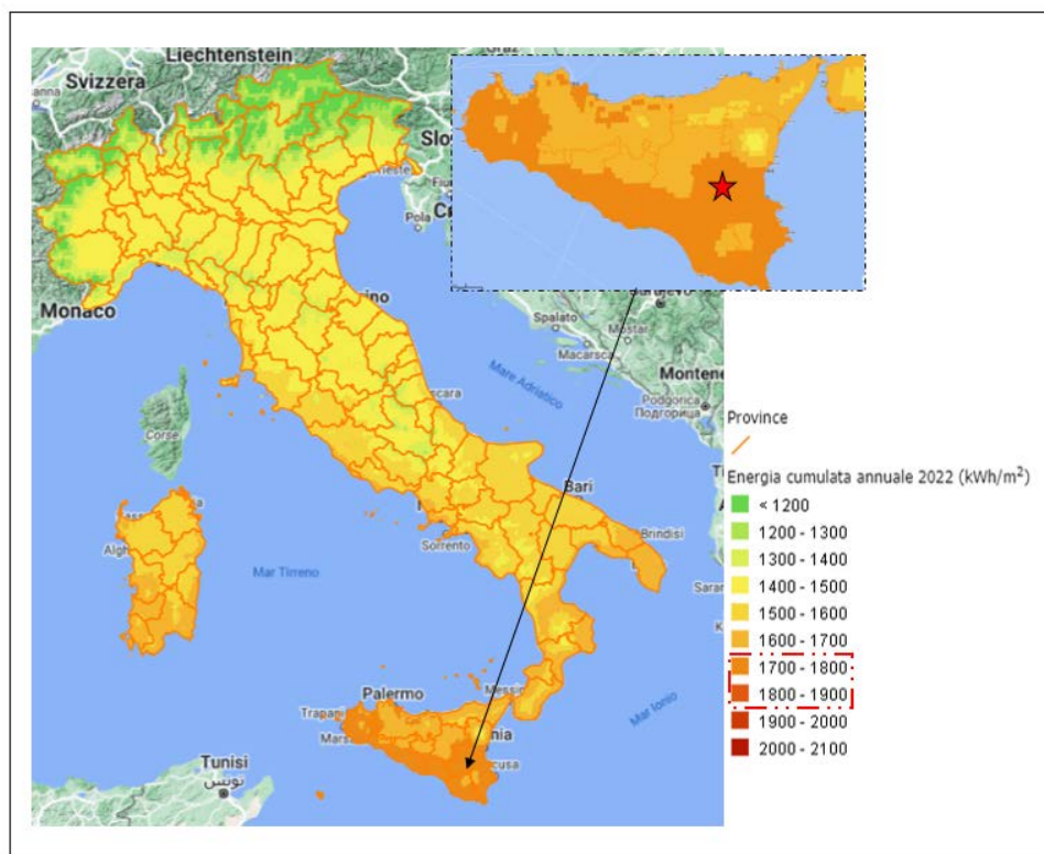
Figura 8: Regime insolazione anno 2022 - Fonte: RSE ( https://sunrise.rse-web.it/ )
