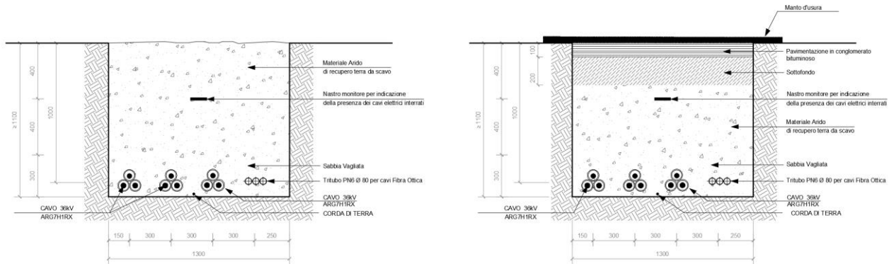
Figura 3.2 – Tipico modalità di posa cavi a 36 kV
