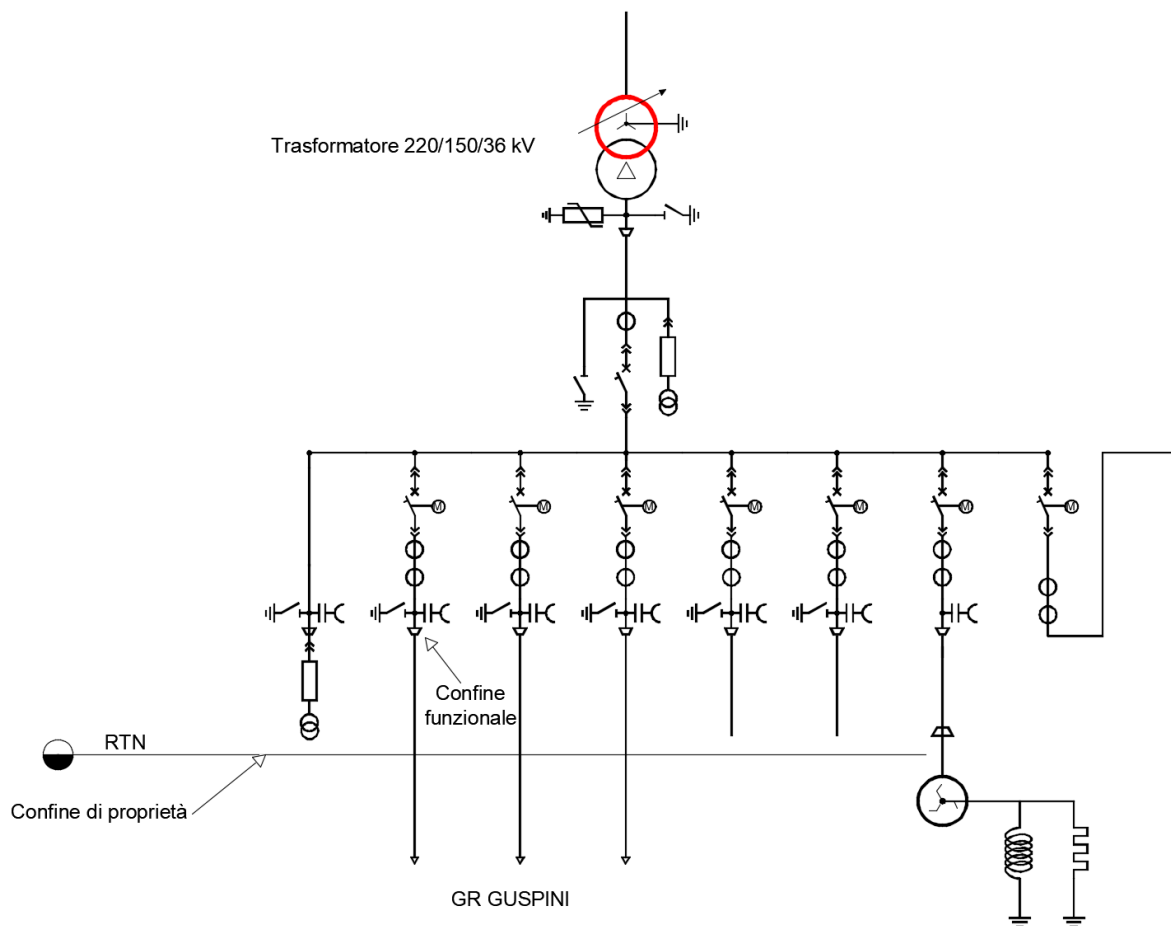
Figura 2.1 – Schema connessione agli stalli di consegna TERNA
