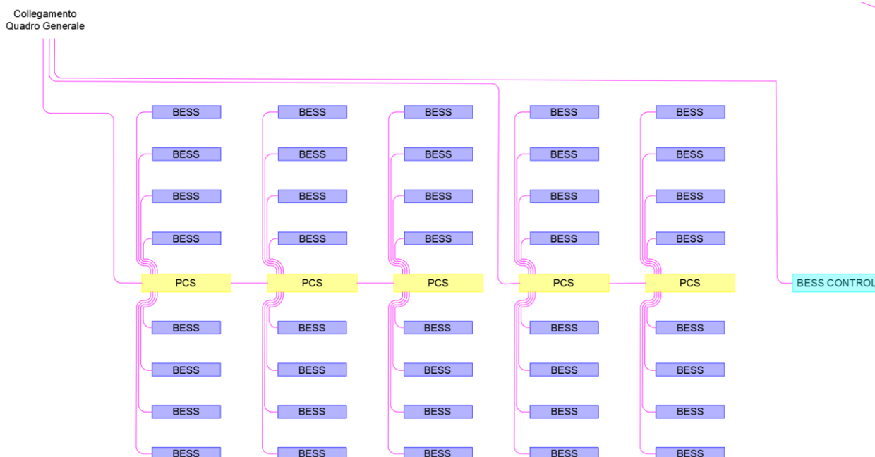
Figura 2.5 – Layout dell'impianto BESS all'interno dell'area disponibile
