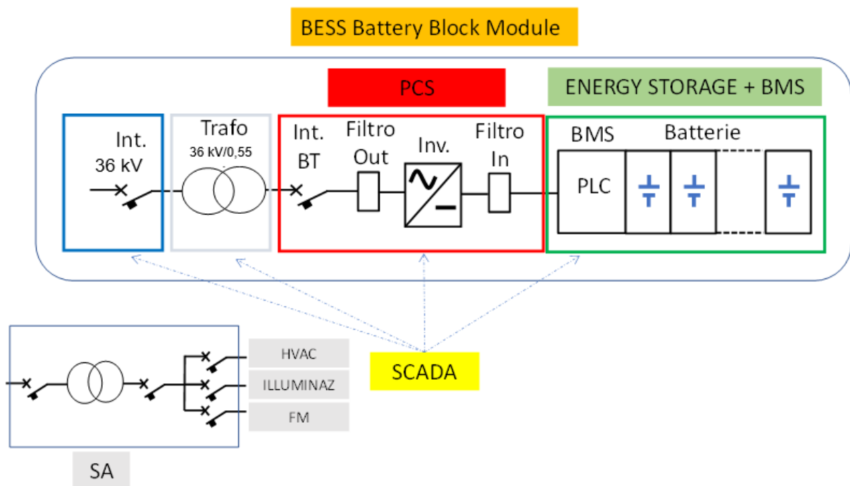
Figura 2.1 - Schema a Blocchi BESS battery block
