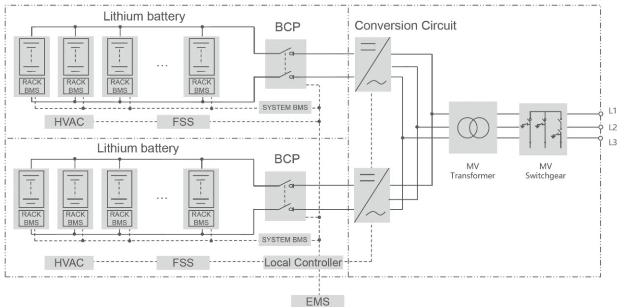
Figura 2.3 – Schema tipologico funzionale singolo battery block
