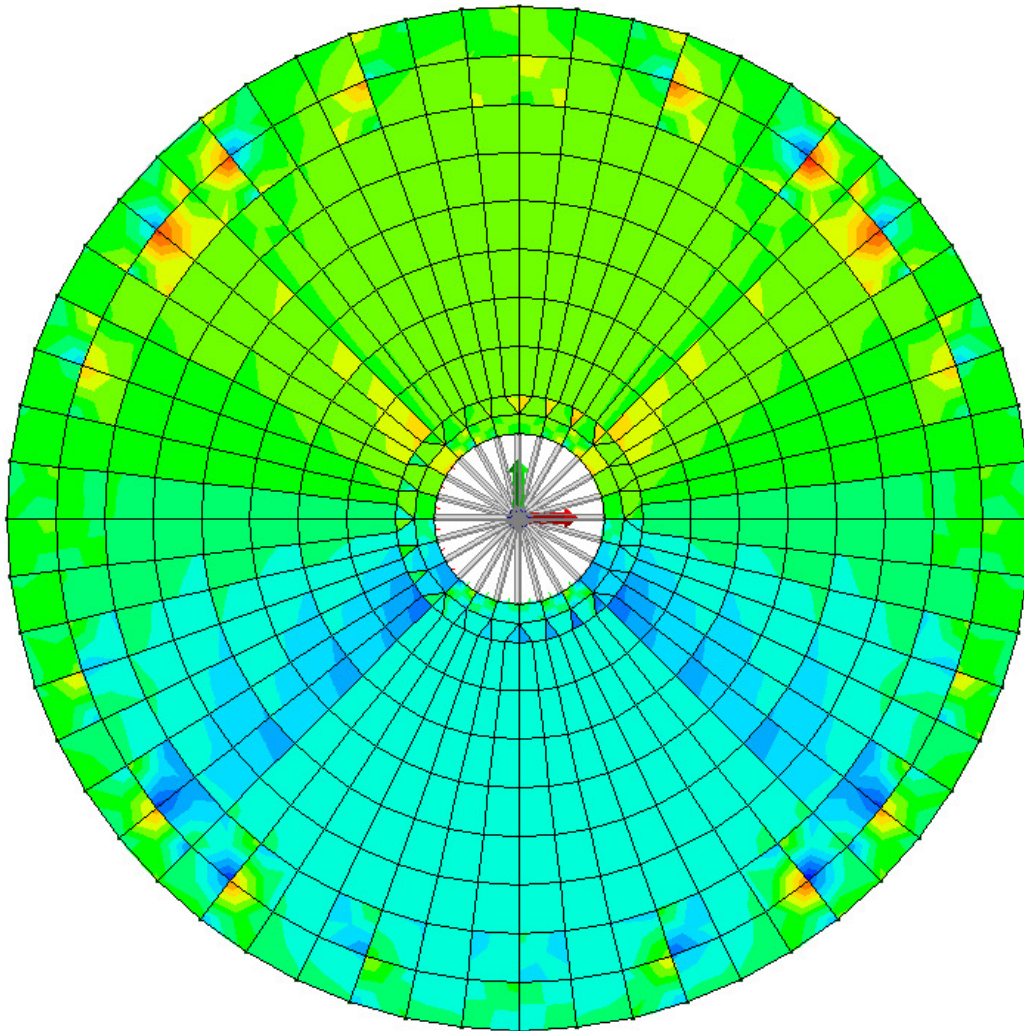
TENSIONE M 1-1
