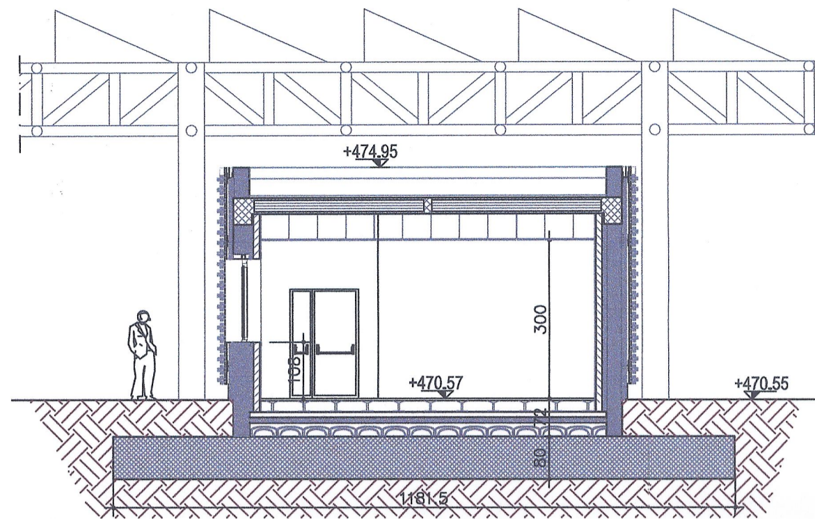
SEZIONE A-A
