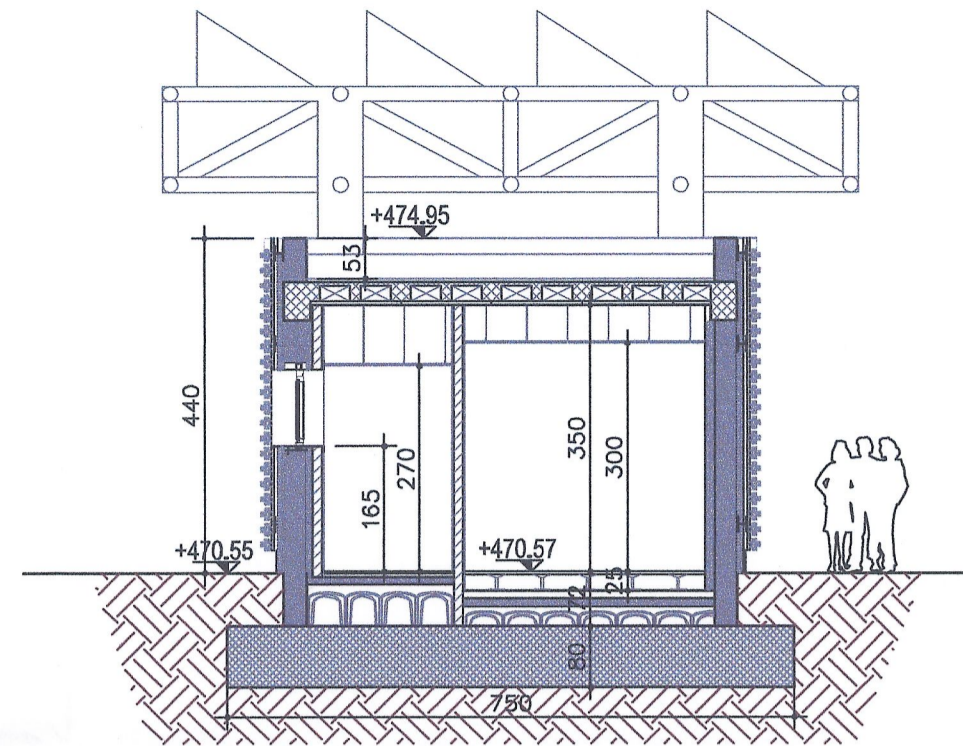
SEZIONE B-B
