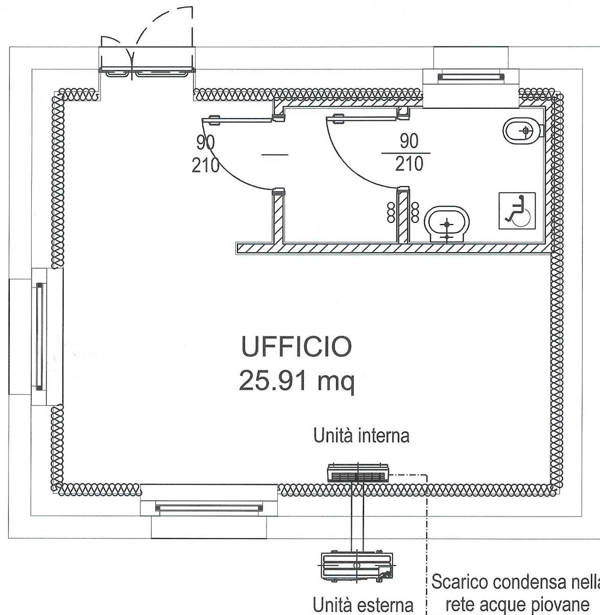
PLANIMETRIA IMPIANTO DI RISCALDAMENTO - SCALA 1:50
