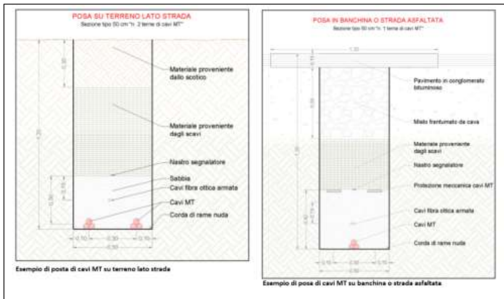
FIGURA 9: ESEMPI DI POSA CAVI
