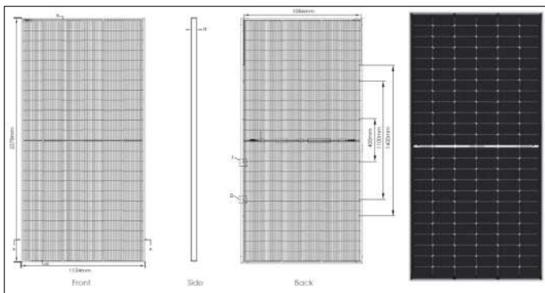
FIGURA 7: PANNELLO FV PARI A 570 WP CON DIMENSIONI 22785 X 1134 X 30 MM
