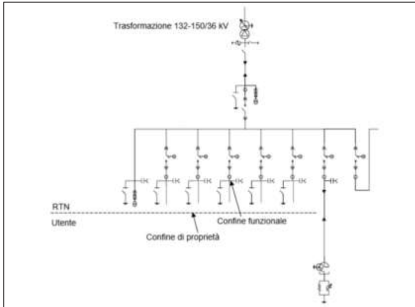
FIGURA 10: SCHEMA DI CONNESSIONE ESEMPLIFICATIVO A 36 kV (ESTRATTO DA GUIDA TERNA)
