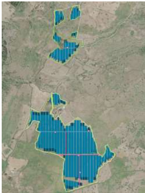
FIGURA 6: LAYOUT DI PROGETTO
