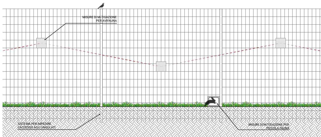
FIGURA 18 – ESEMPIO RECINZIONE METALLICA CHE DELIMITA L'AREA DI PERTINENZA DELL'IMPIANTO
