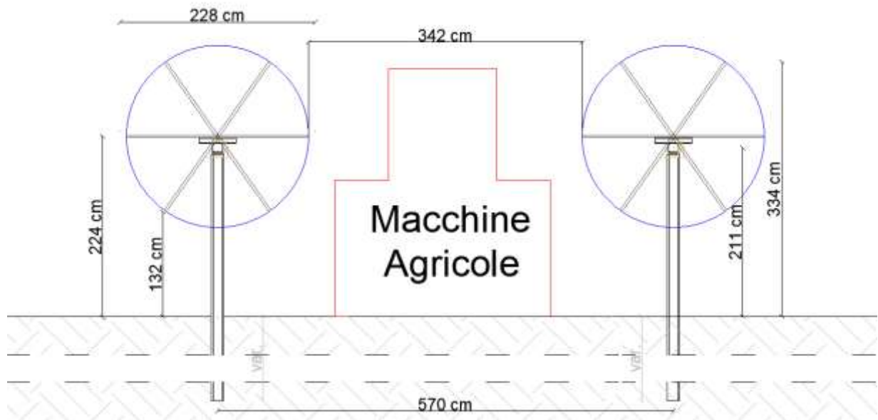
FIGURA 4: CONFIGURAZIONE TRACKER IMPIANTO AGRIVOLTAICO
