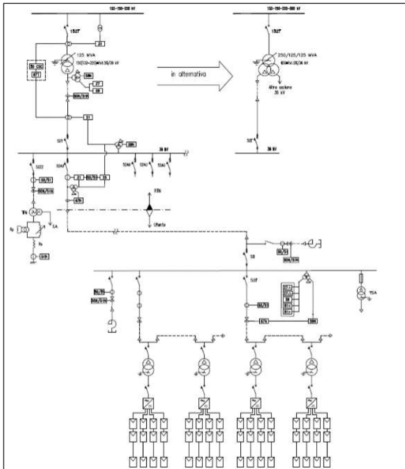
FIGURA 11: ASSETTO DELLE PROTEZIONI CONTRO I GUASTI E LE PERTURBAZIONI NELLA RETE DI UNA CENTRALE FOTOVOLTAICA (ESTRATTO DA ALLEGATO A.68 DEL 19 MAGGIO 2022)
