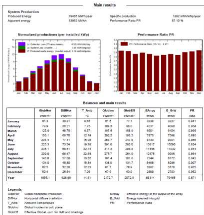
FIGURA 5: PRODUCIBILITA' ELETTRICA DELL'IMPIANTO AGRIVOLTAICO VALUTATA TRAMITE PVSYST
