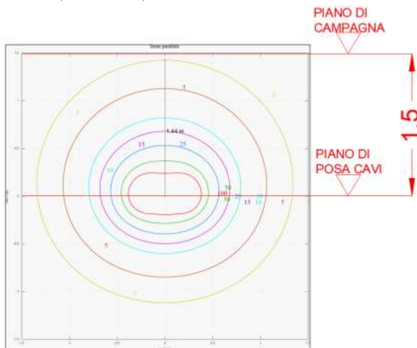
FIGURA 2: CURVE ISOINDUZIONE – 3 LINEE AT INTERRATE
