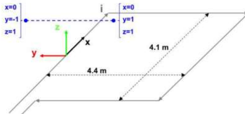
Fig. 9: Schema di spira quadrata.
