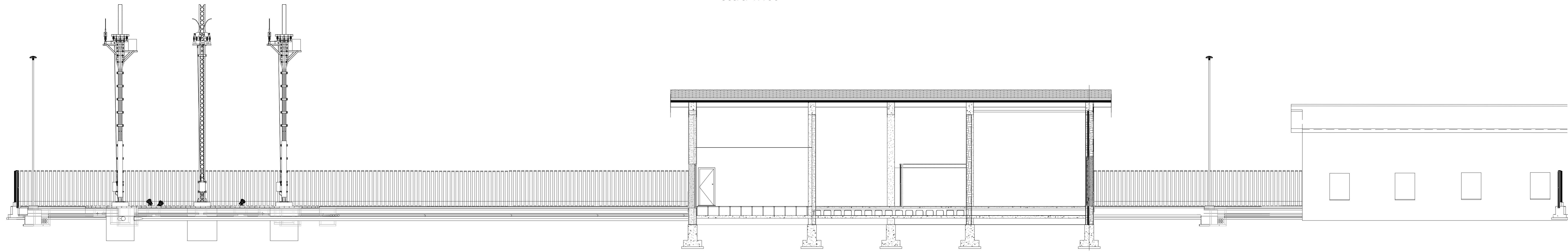
SEZIONE B-B scala 1:100
