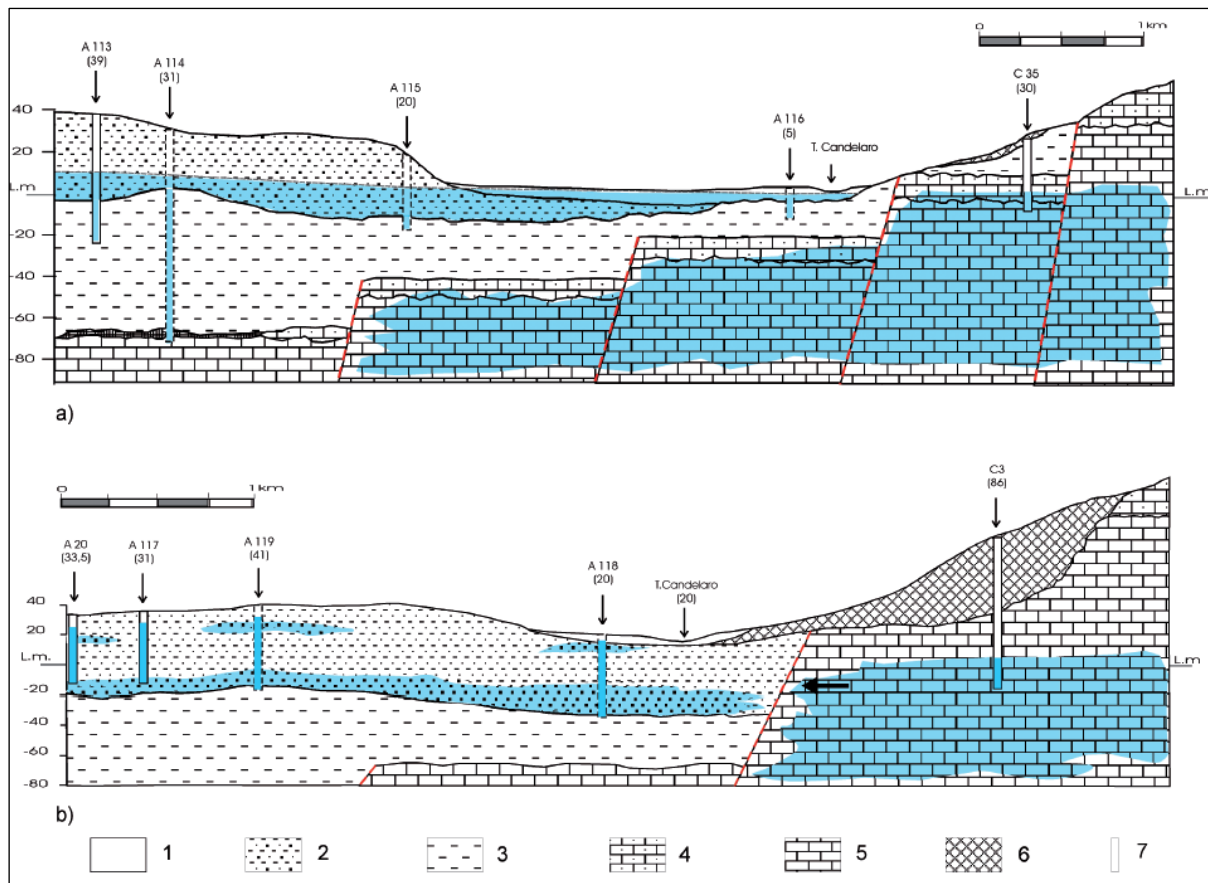
Figura 4.2: Sezioni idrogeologiche. Legenda 1) Depositi d'alveo (Olocene); 2) depositi della pianura alluvionale (Olocene – Pleistocene sup.); 3) argille grigio- azzurrognole con intercalazioni sabbiose (Pleistocene inf. – Pliocene sup.) 4) Calcarenite (Pliocene sup. – Miocene); calcari della piattaforma carbonatica apula (Cretaceo); 6) Conoidi detritiche (Olocene – Pleistocene sup.) 7) Pozzo (in tratteggio, se proiettato).
