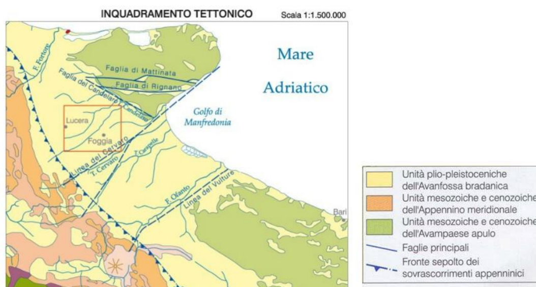
Figura 3.4: Schema geologico e strutturale dell'area del Tavoliere e del Subappennino Dauno.
