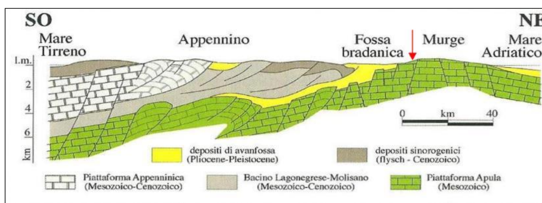
Figura 3.5: Sezione geologica schematica attraverso l'avanfossa appenninica.
