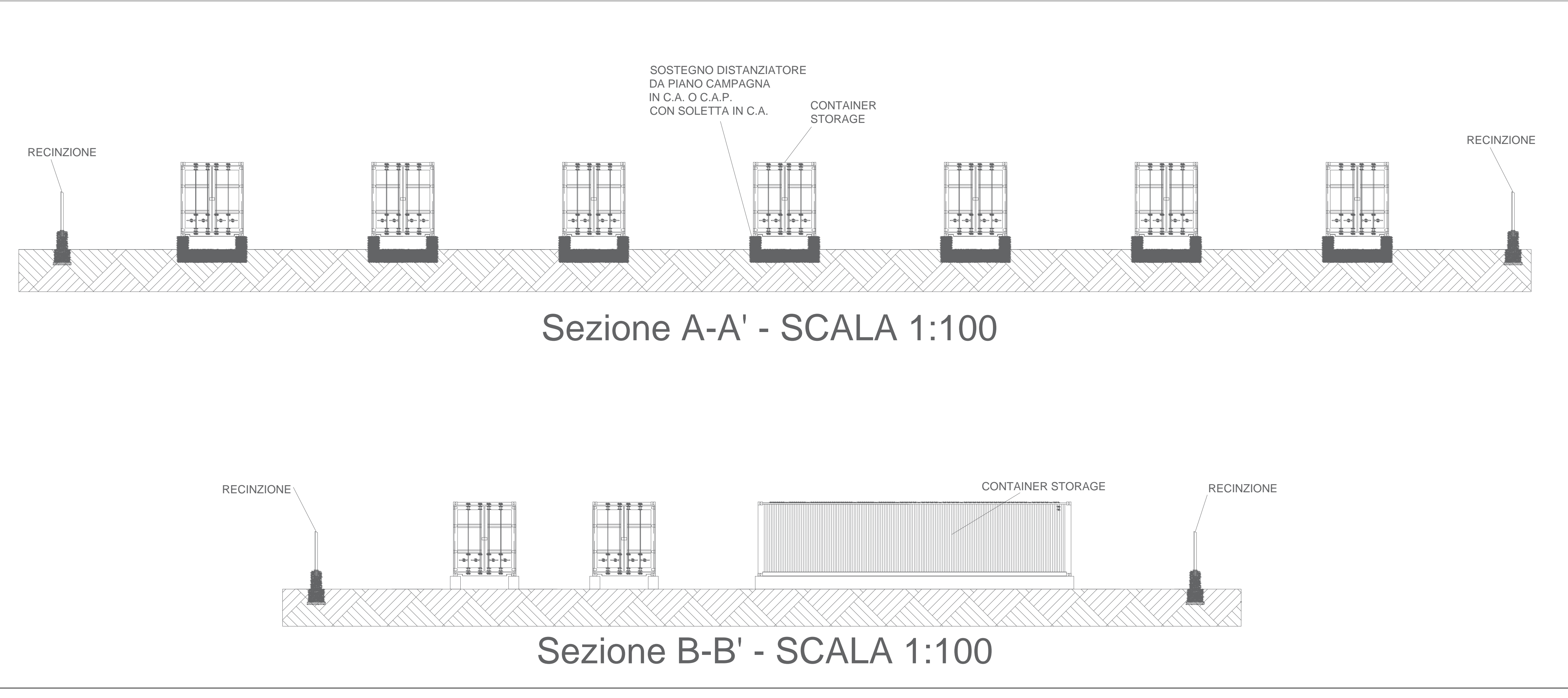
PARTICOLARE SEZIONI - SCALA 1:100
