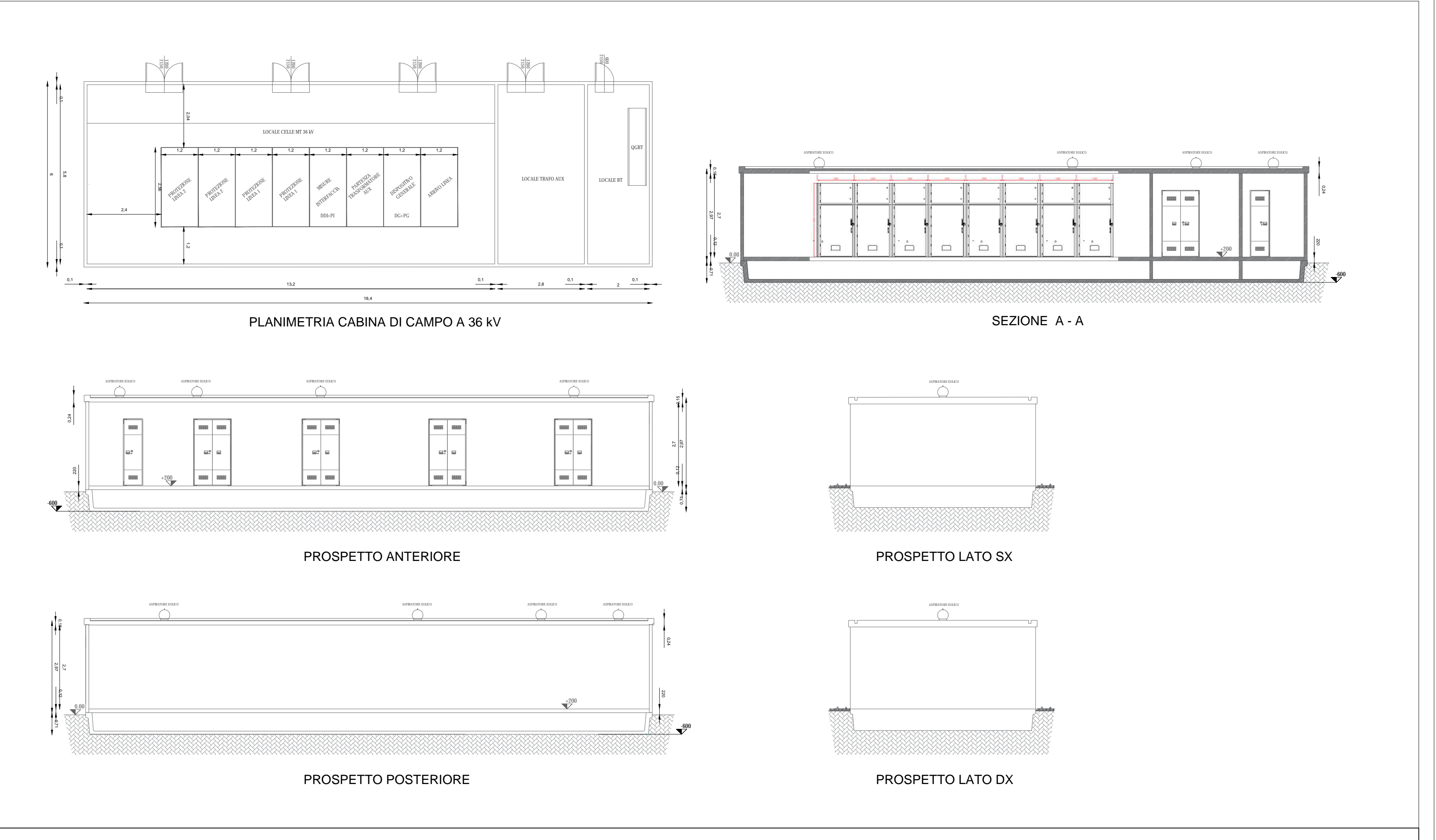
PARTICOLARE CABINA - SCALA 1:100
