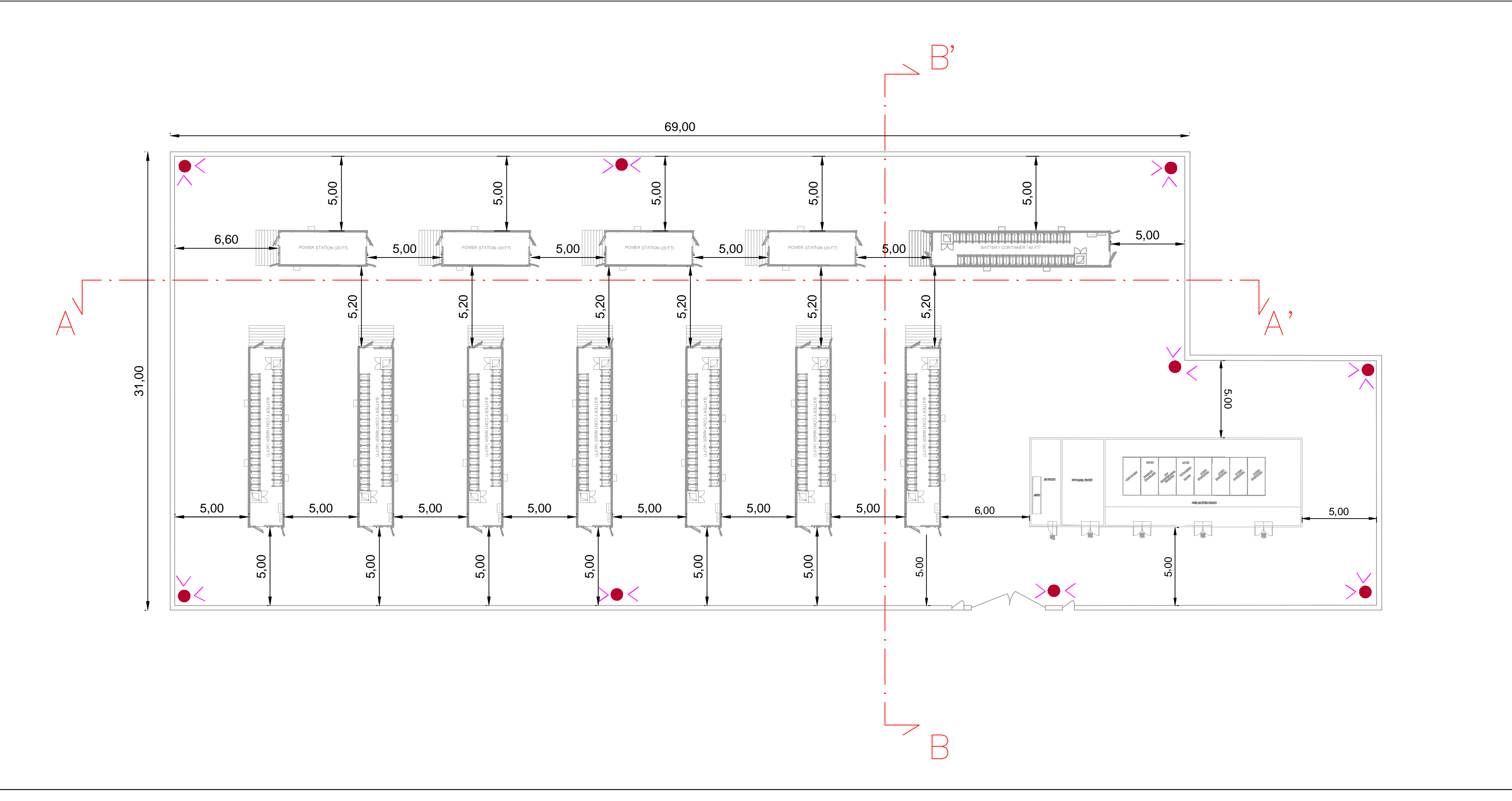
PARTICOLARE AREA STORAGE - SCALA 1:200
