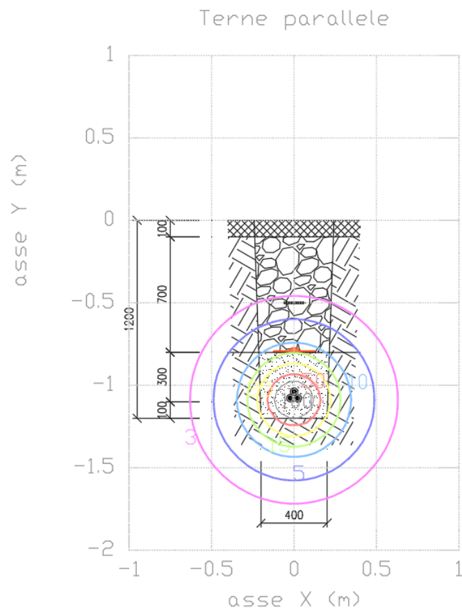
Figura 2 – Livelli di campo magnetico per il solo cavidotto B
