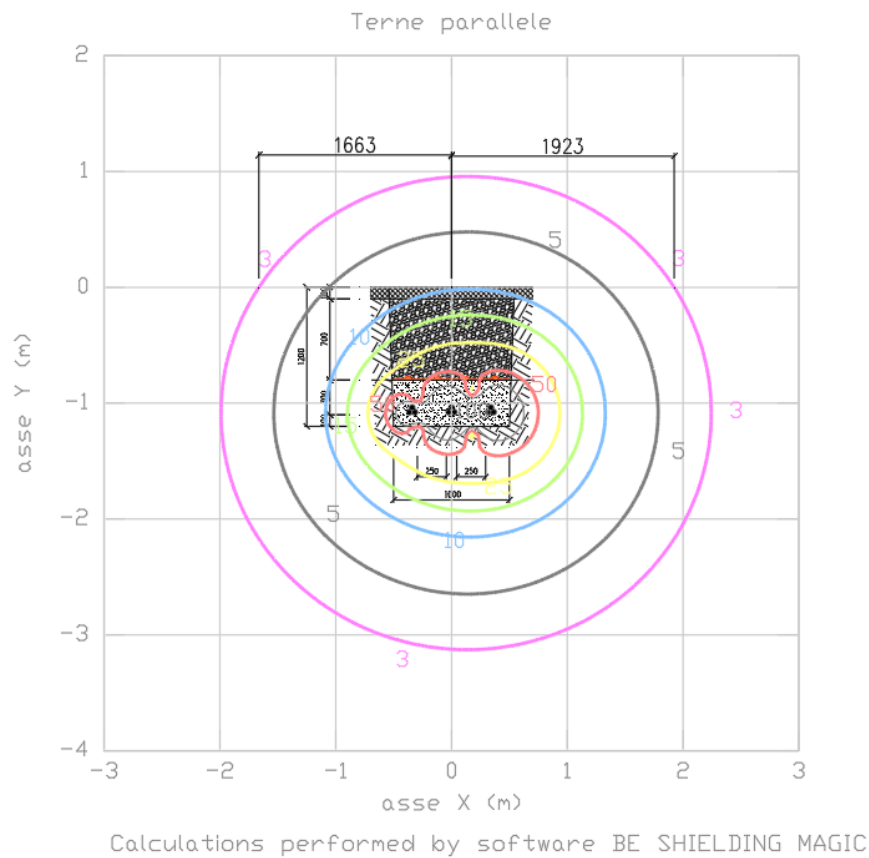
Figura 3 – Livelli di campo magnetico per il tratto in cui i cavidotti A e B sono interrati nel medesimo scavo
