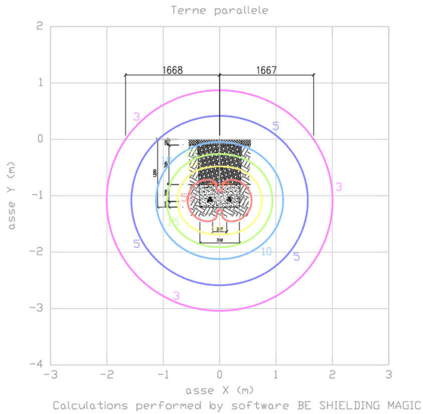
Figura 1 – Livelli di campo magnetico per il solo cavidotto A
