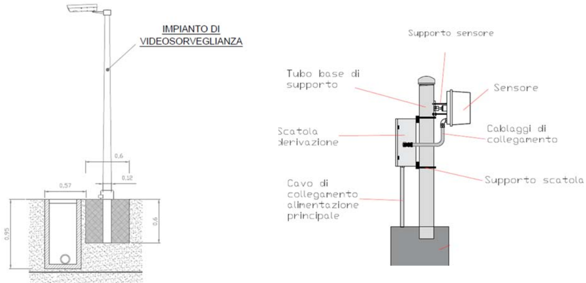
Fig. 21 – Sistema antintrusione
