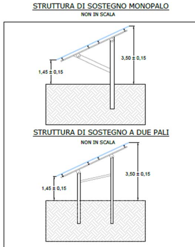
Fig. 2 - Struttura di supporto moduli
