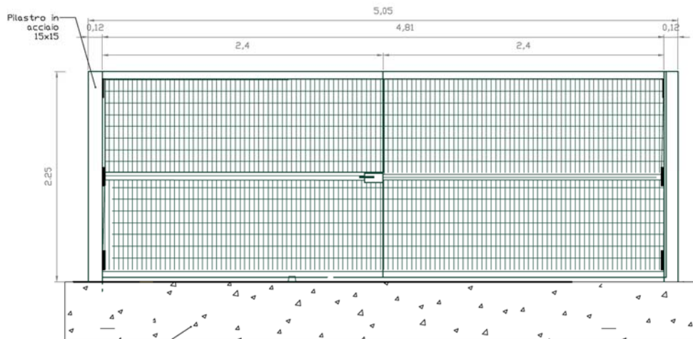
Fig. 19 – Cancello a doppia anta
