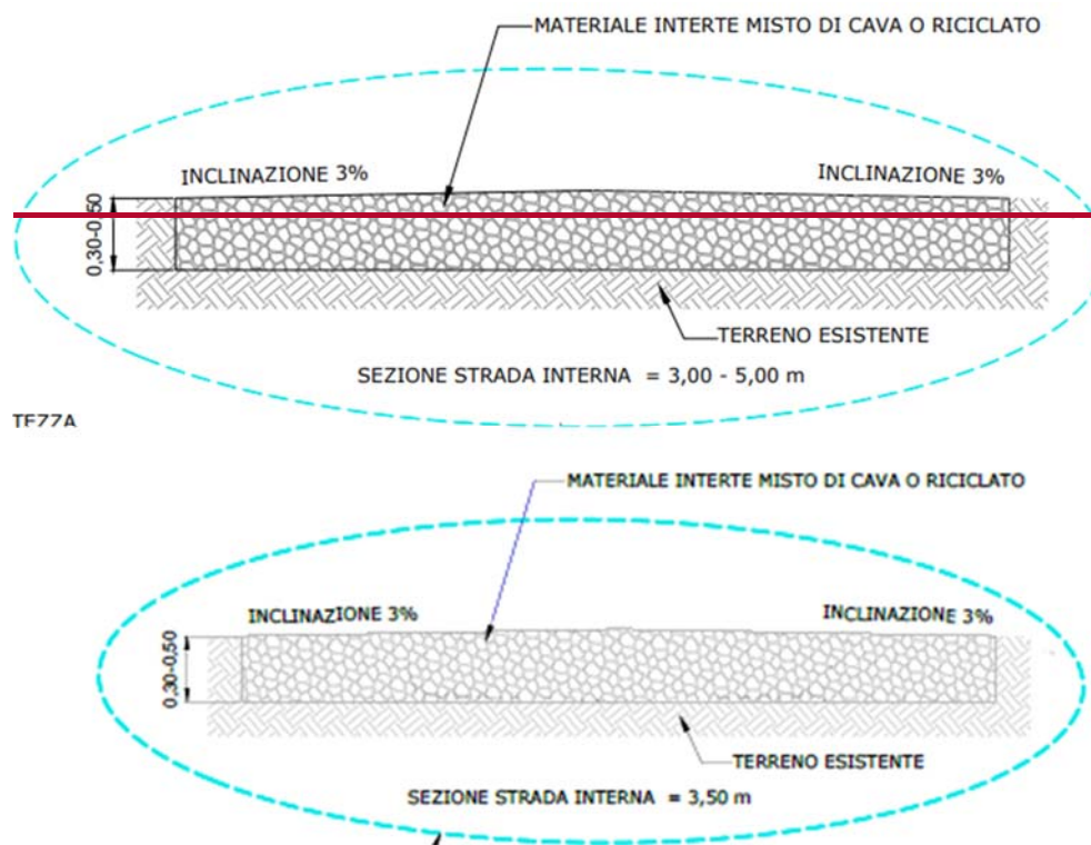
Fig. 20 – Sezione strada perimetrale
