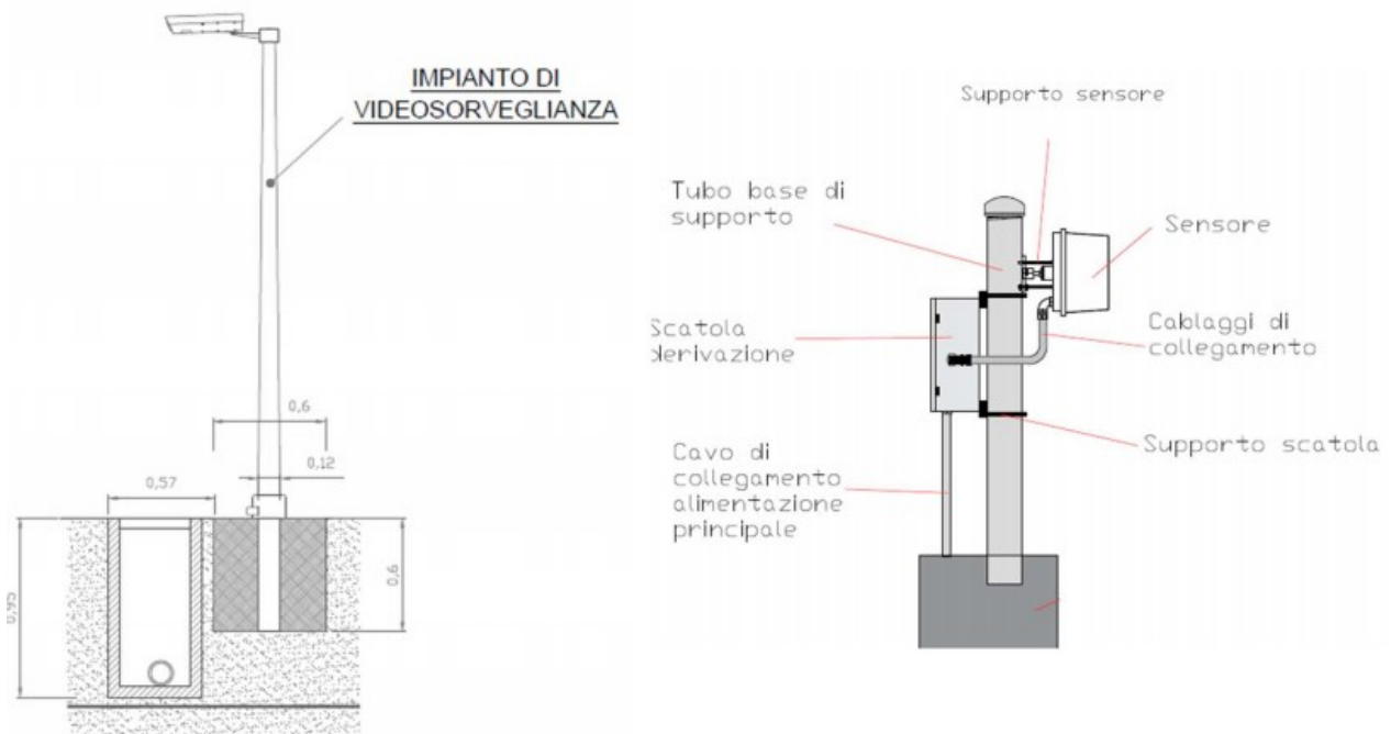
Figura 5-5: Sistema antintrusione
