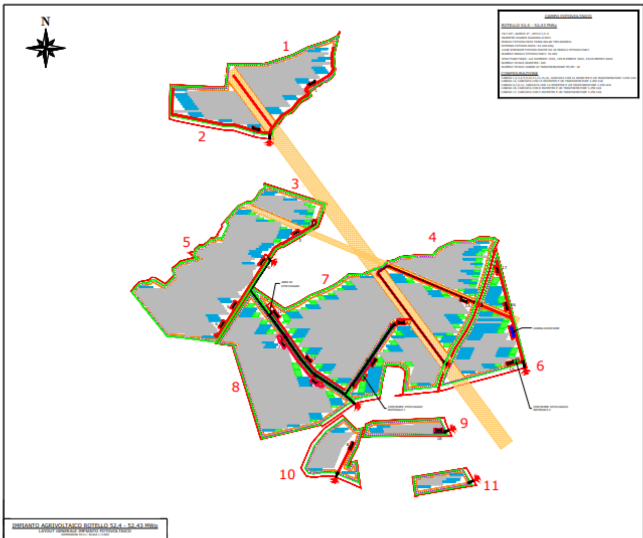
Figura 5-1: Layout impianto
