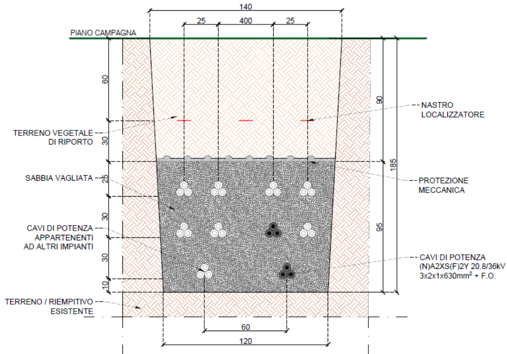
Figura 10: Sezione tipica di scavo tratto in condivisione con altri cavidotti
