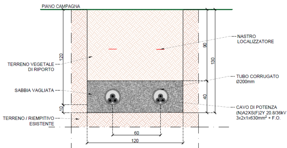
Figura 11: Sezione tipica di scavo tratto terminale per collegamento in stazione elettrica
