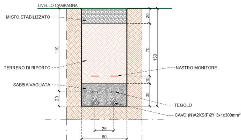
Figura 8: Sezione di scavo cavidotto AC AT
