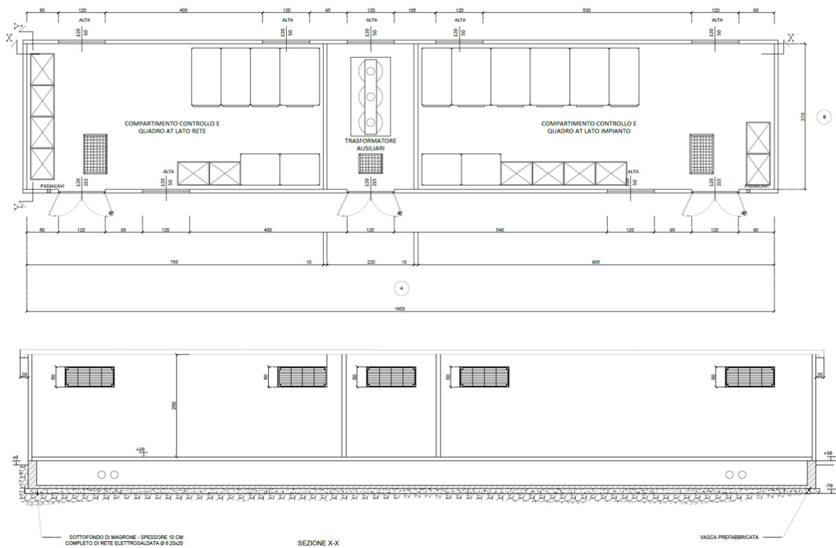
Figura 6: Pianta, Prospetti e Sezioni Cabina di Raccolta
