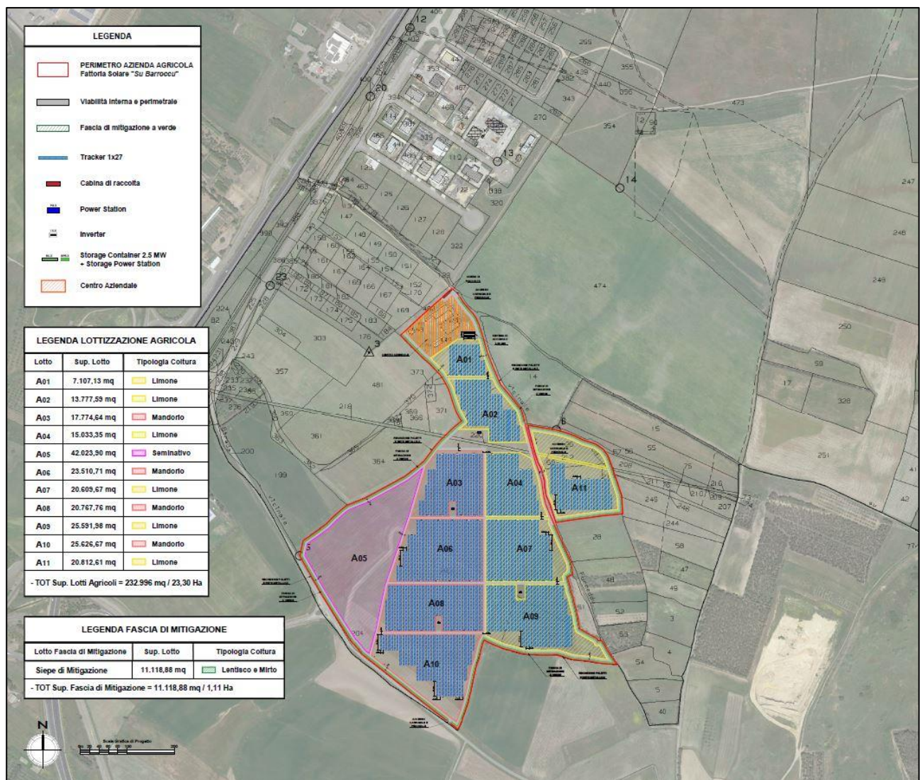
Figura 6: Divisione in parcelle e relative superfici utilizzate. Riferimento Elaborato Grafico "2103_T.P.10_Layout Piano Agronomico_Rev00"
