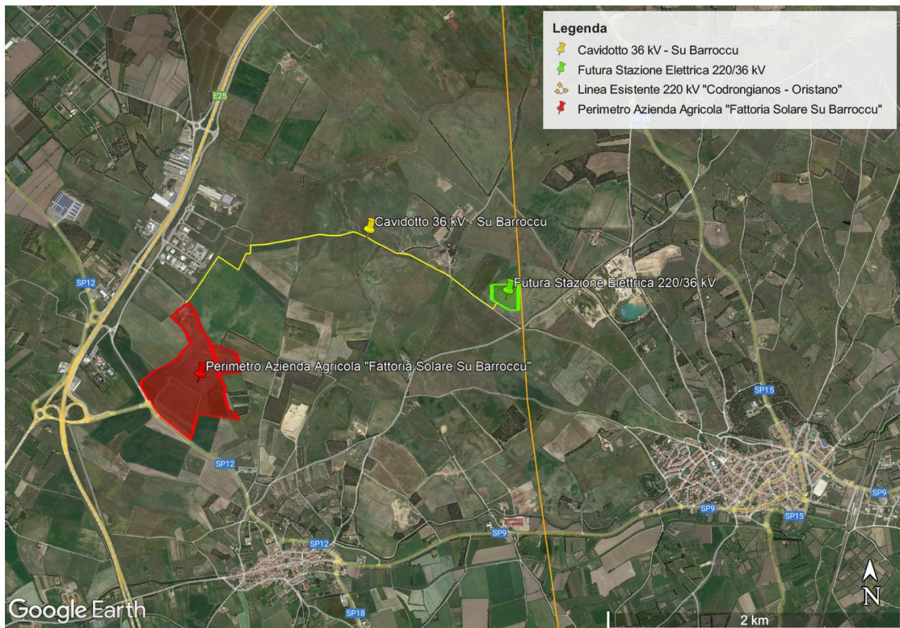
Figura 1: Ubicazione su ortofoto dell'impianto agrivoltaico e delle opere di rete.
