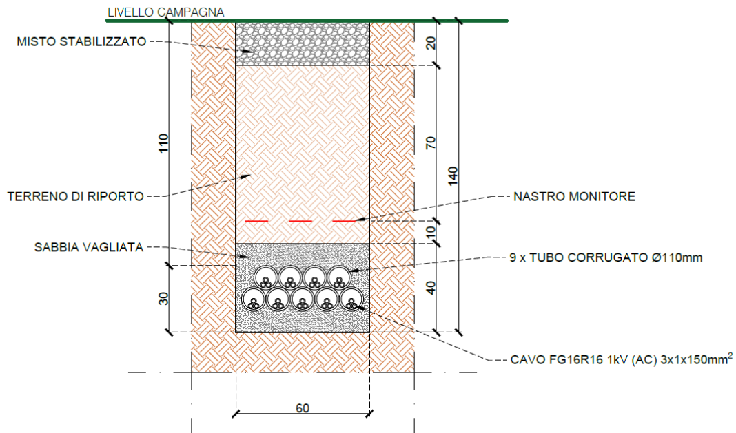
Figura 6: Sezione di scavo tipico
