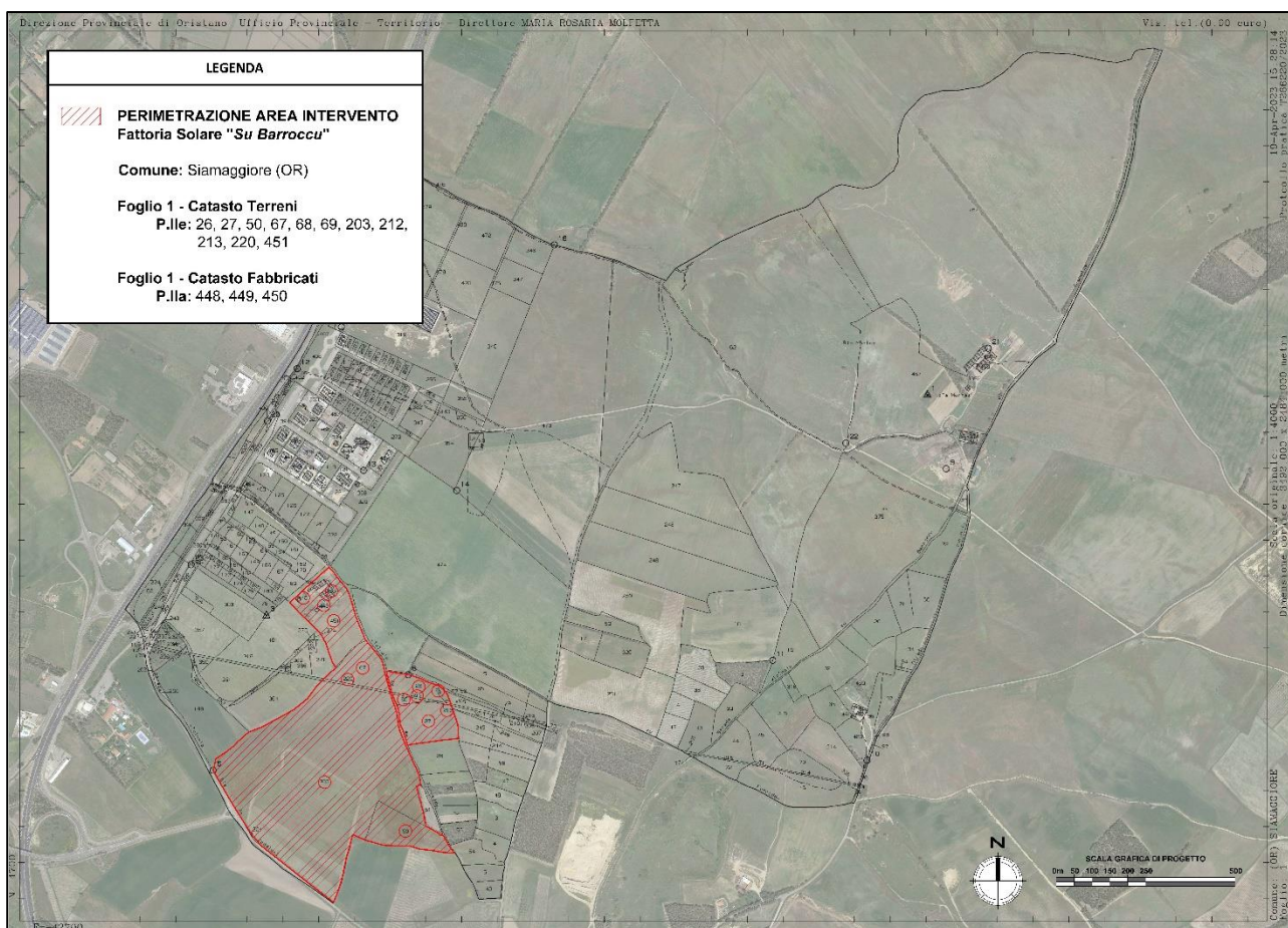
Figura 10: Inquadramento Territoriale Area Impianto su Ortofoto Catastale. Riferimento Elaborato Grafico "2103_T.A.03_Inquadramento Territoriale su Orto-Catastale_Rev00"
