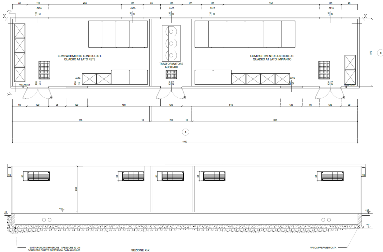
Figura 4: Dettaglio cabina di raccolta
