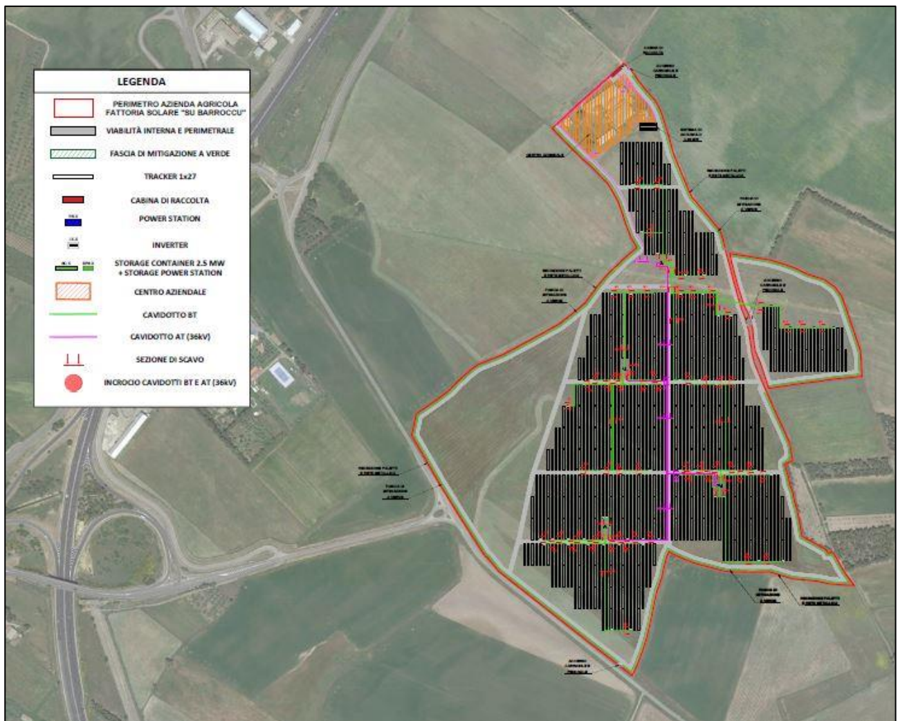
Figura 29: Layout impianto con cavidotti e sezioni di scavo Riferimento Elaborato Grafico "2103_T.P.07_Layout Impianto con cavidotti e sezioni di scavo_Rev00"
