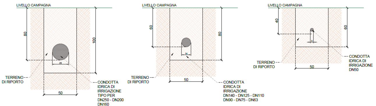
Figura 8: Sezione di scavo condotte idriche
