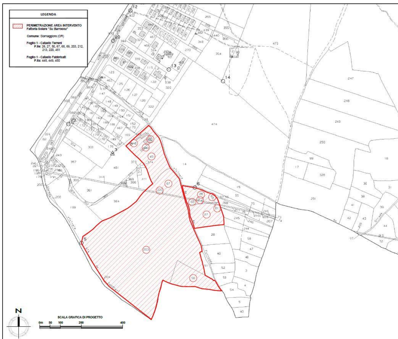
Figura 9: Inquadramento Territoriale Catastale Area Impianto Agrivoltaico. Riferimento Elaborato Grafico "2103_T.A.04_Inquadramento Territoriale su Catastale_Rev00"
