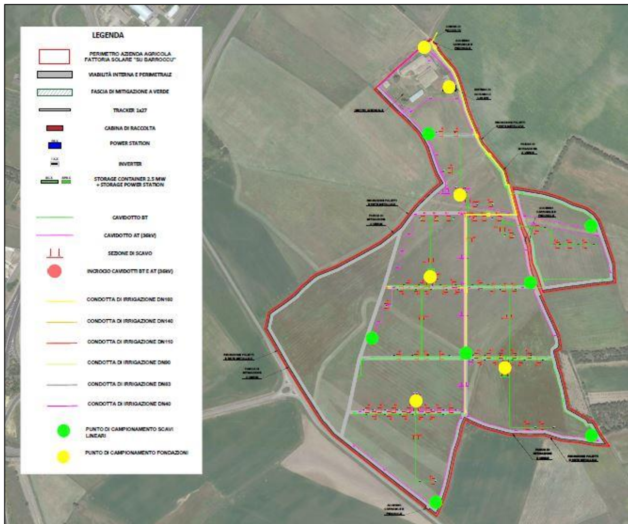
Figura 31: Layout impianto con piano di campionamento
