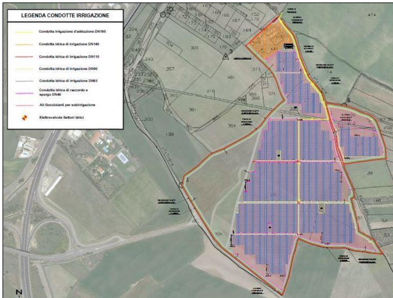
Figura 30: Layout impianto di irrigazione e fertirrigazione Riferimento Elaborato Grafico "2103_T.P.11_Layout Impianto Irrigazione-Fertirrigazione_Rev00"
