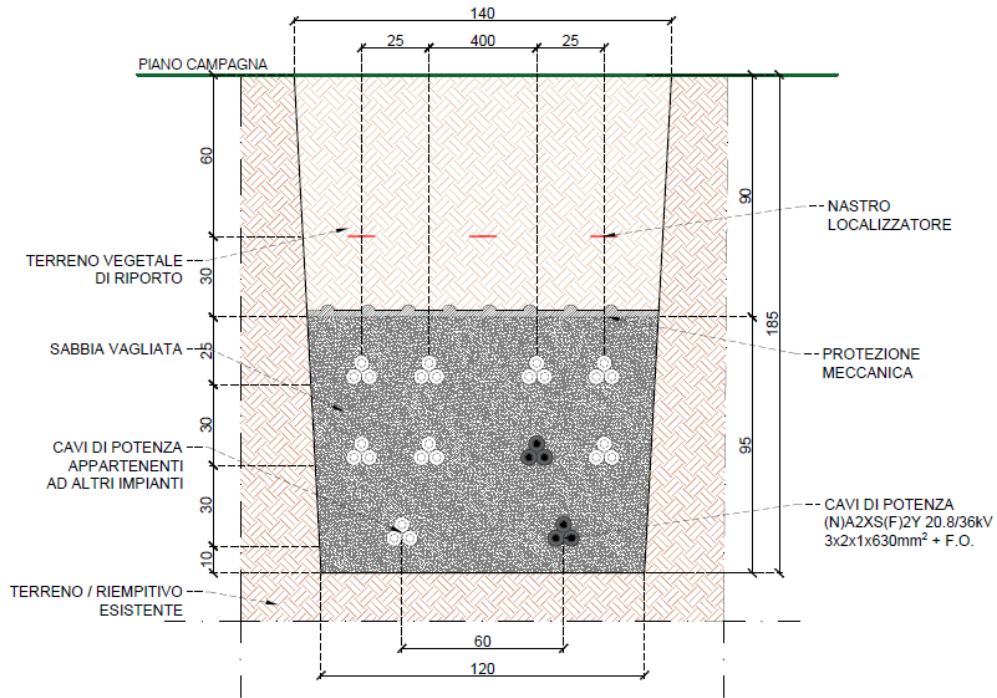
Figura 7: Sezione di scavo cavidotto AT
