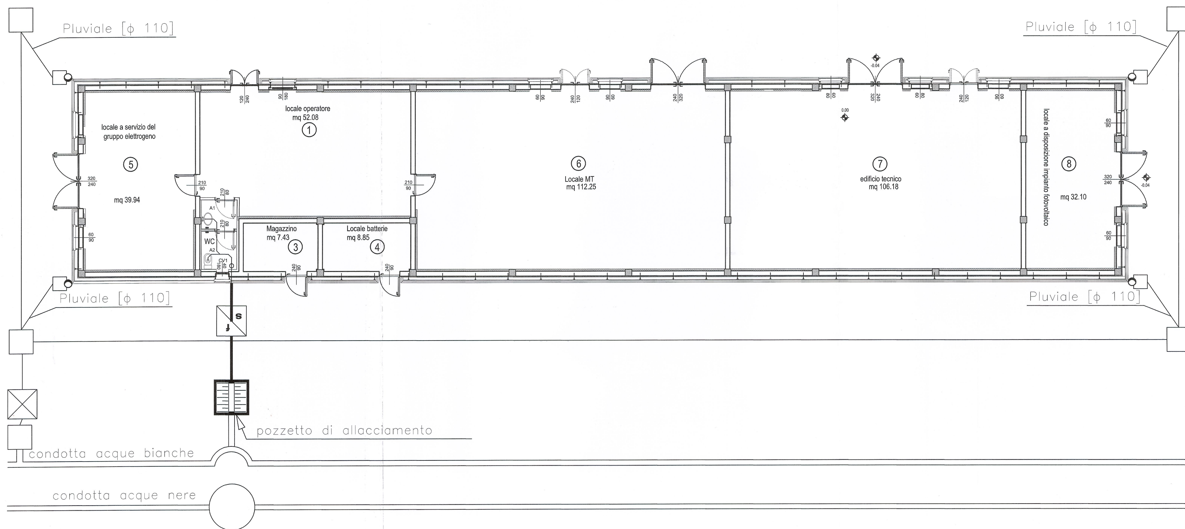
PLANIMETRIA IMPIANTO DI SCARICO - SCALA 1:100
