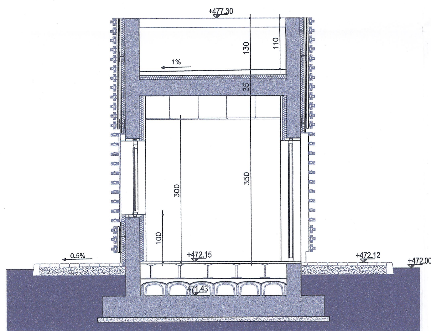
SEZIONE A-A
