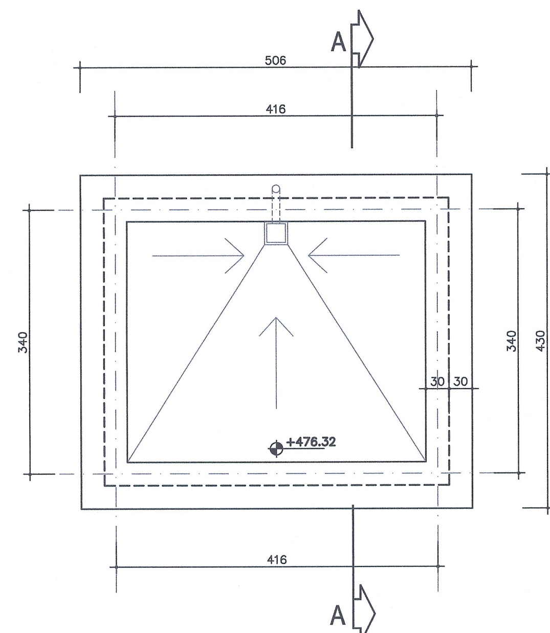
PIANTA COPERTURA
