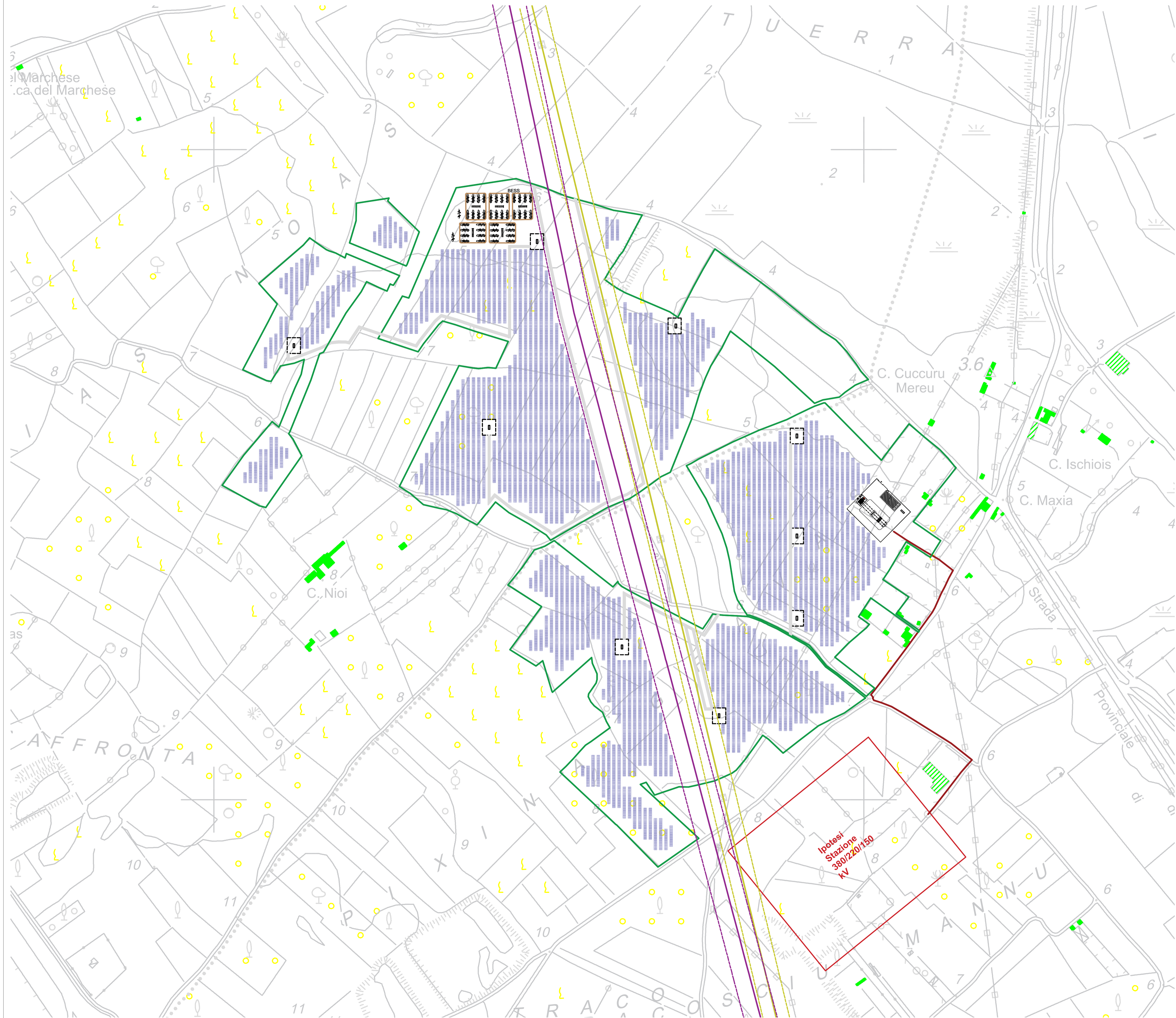
PLANIMETRIA - INQUADRAMENTO AREA DI PROGETTO CON LINEE ELETTRICHE EFASCE DI RISPETTO SU BASE CTR
