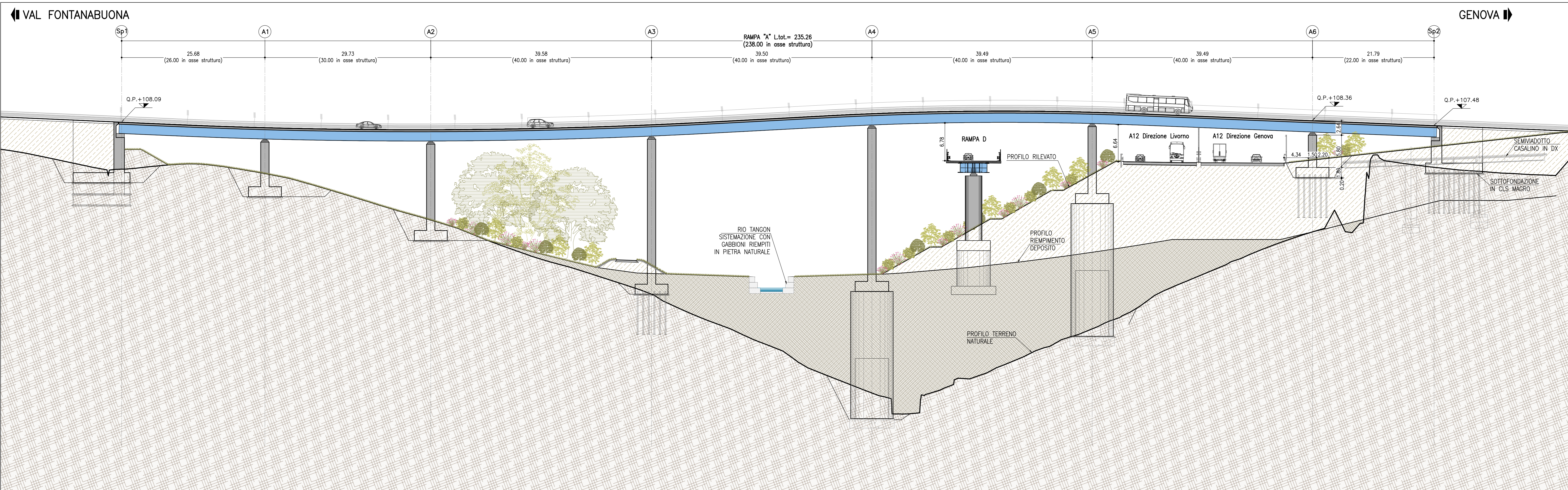
Prospetto A-A' (lato sud) - Scala 1:300
